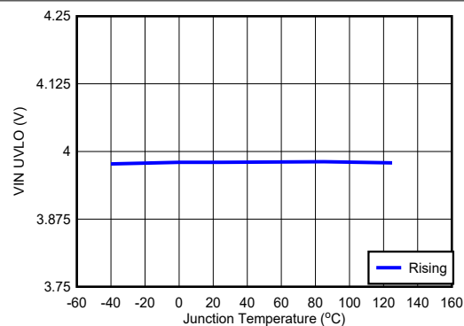
图 5-8. Vin UVLO
