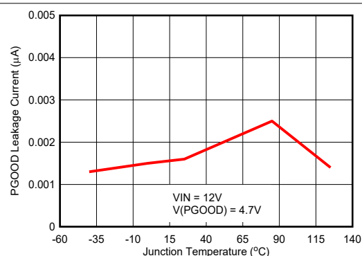
图 5-10. PG Leakage
