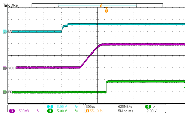
图 7-11. EN Start-Up - With Load
