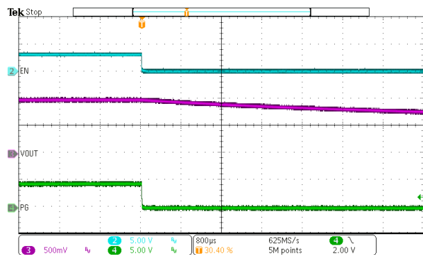
图 7-10. EN Shutdown No Load
