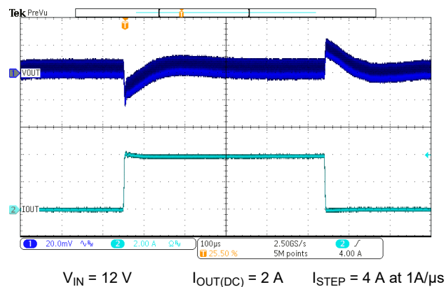
图 7-8. Load Transient
