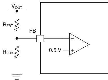
图 6-3. FB Resistor Divider
