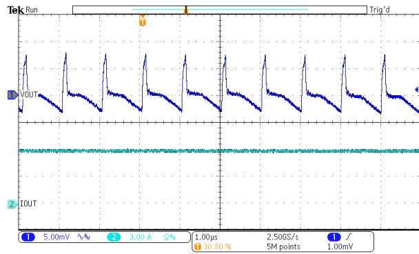
图 7-16. Output Ripple – 6A Load
