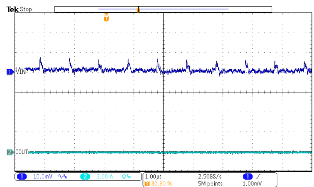
图 7-17. Input Ripple – No Load
