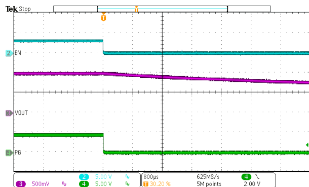
V_{IN} = 12V I_{OUT} = 0A 图 7-10. EN Shutdown No Load
