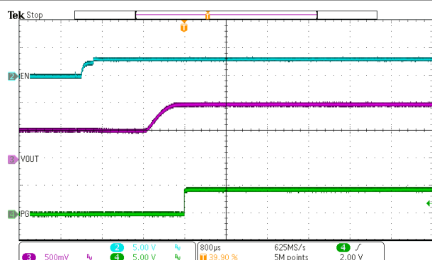
V_{IN} = 12V I_{OUT} = 0A 图 7-12. EN Start-Up – 0.5V Prebias
