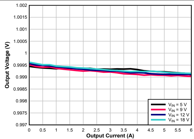
图 7-5. Load Regulation
