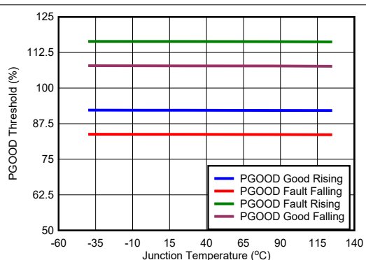
图 5-9. PG Threshold
