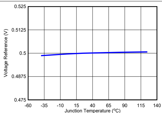
图 5-7. Voltage Reference
