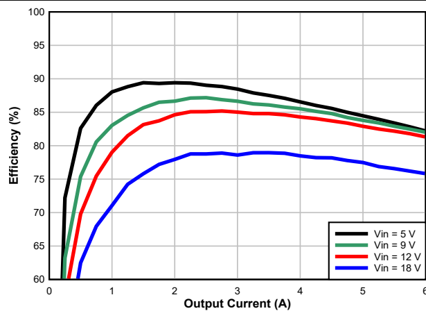
图 7-4. Efficiency
