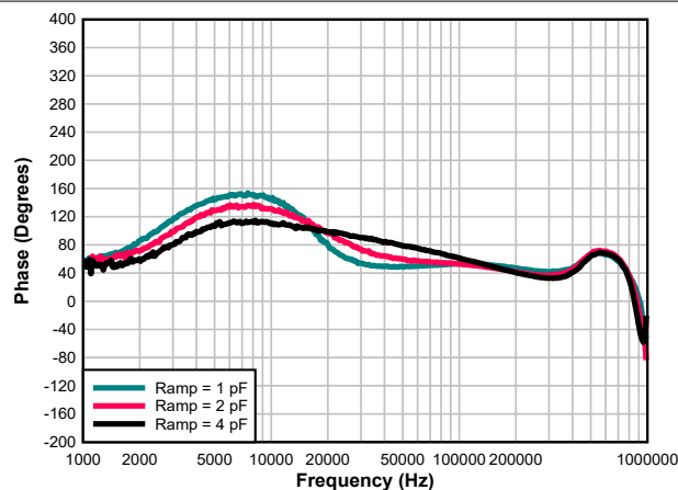
图 6-7. Loop Phase vs Ramp Settings
