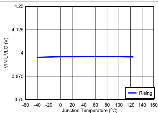
图 5-8. Vin UVLO
