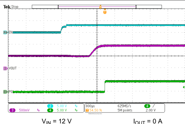
图 7-12. EN Start-Up - 0.5-V Prebias
