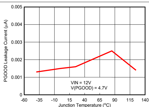
图 5-10. PG Leakage
