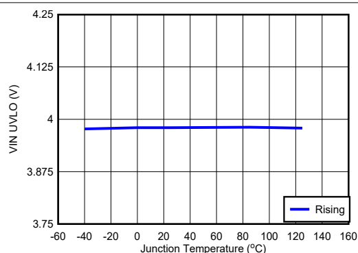
图 5-8. Vin UVLO
