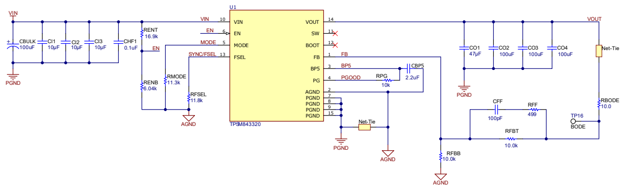
图 7-1. 12-V Input, 1.0-V Output, 1-MHz Schematic
