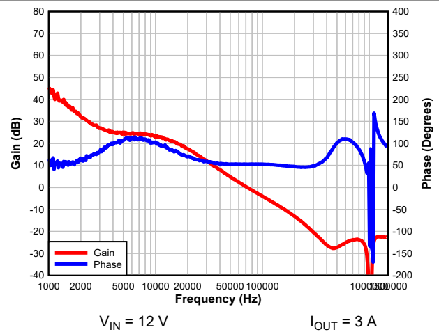
图 7-7. Bode Plot
