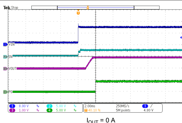
图 7-13. VIN Start-Up
