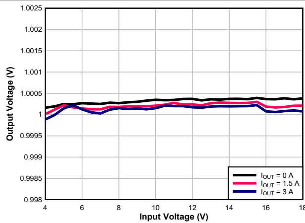
图 7-6. Line Regulation
