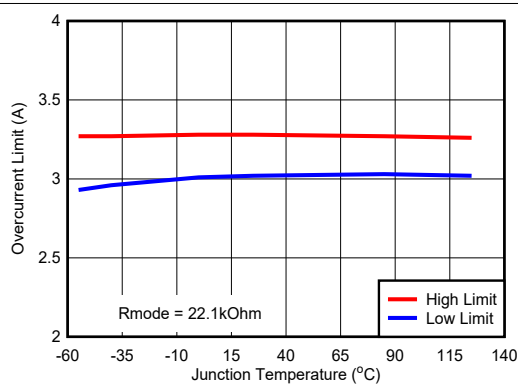
图 5-4. Overcurrent Limit : R = 22.1kOhm
