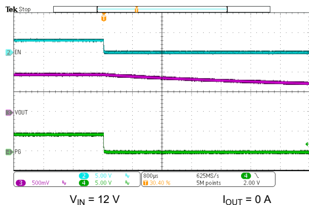
图 7-10. EN Shutdown No Load
