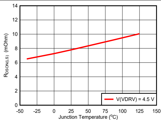
图 5-2. Low-Side FET Rdson
