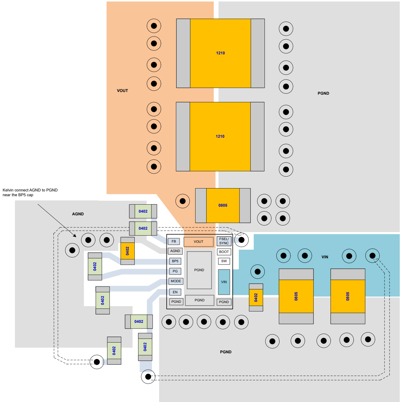
图 7-19. Example PCB Layout
