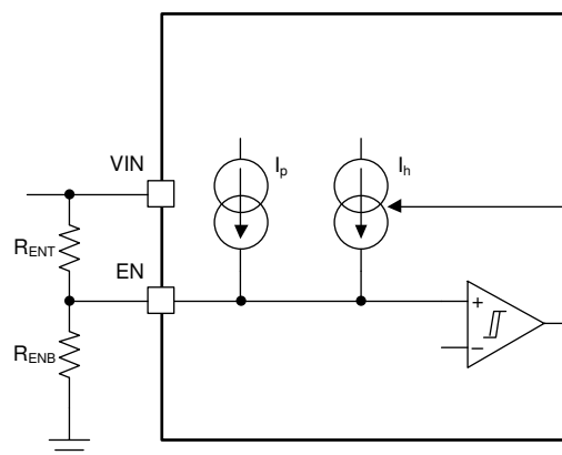
图 6-2. Adjustable UVLO Using EN
