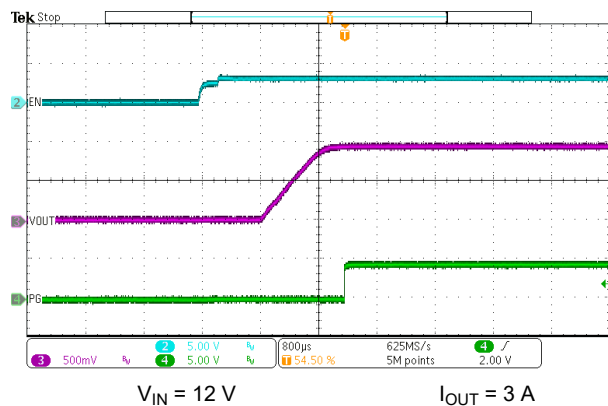
图 7-11. EN Start-Up - With Load
