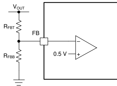
图 6-3. FB Resistor Divider
