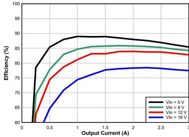
图 7-4. Efficiency
