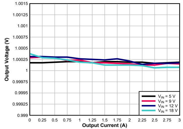
图 7-5. Load Regulation
