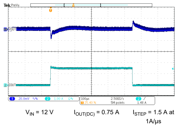
图 7-8. Load Transient
