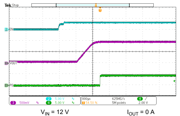
图 7-9. EN Start-Up - No Load
