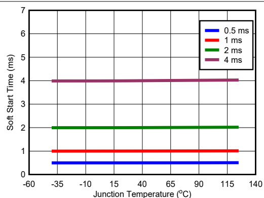
图 5-11. Soft Start
