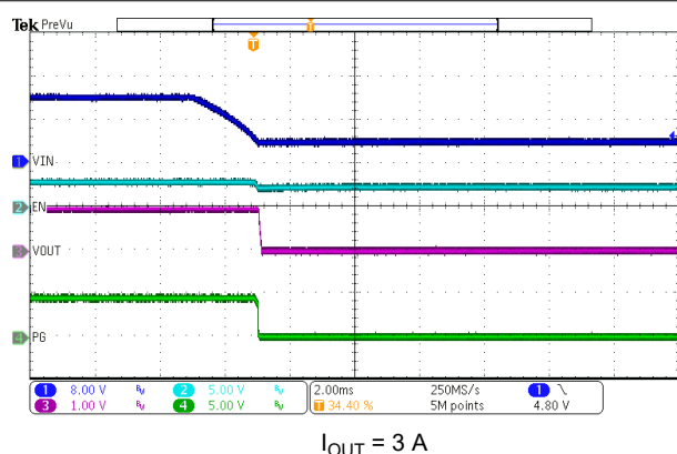
图 7-14. VIN Shutdown
