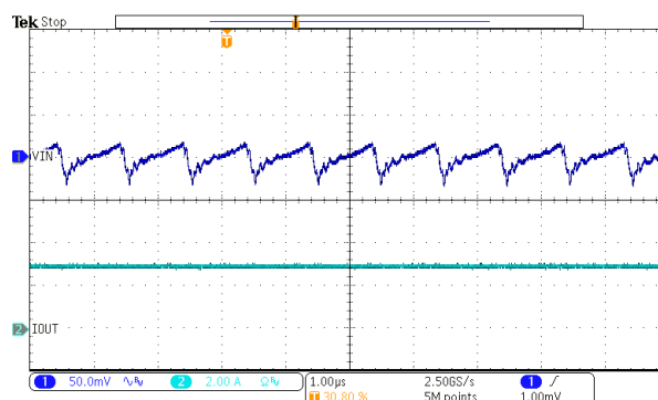
图 7-16. Output Ripple – 3-A Load
