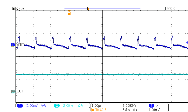
图 7-16. Output Ripple – 3-A Load
