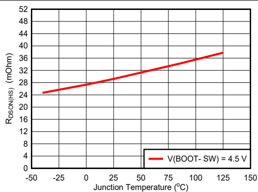
图 5-1. High-Side FET Rdson
