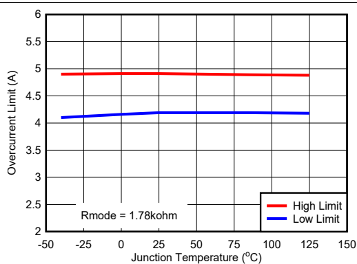
图 5-3. Overcurrent Limit : R = 1.78kOhm
