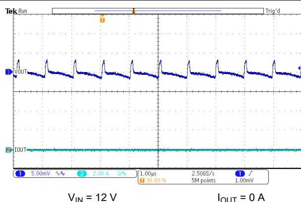
图 7-15. Output Ripple - No Load
