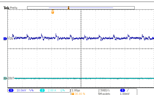
图 7-17. Input Ripple – No Load
