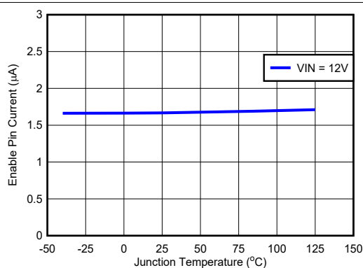
图 5-6. Enable Pin Current
