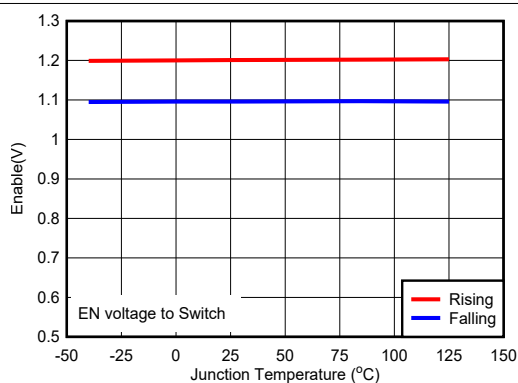
图 5-5. Enable Voltage
