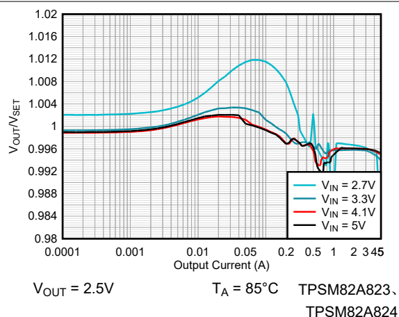
图 8-17. VOUT 精度
