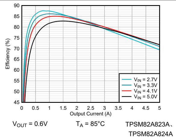
图 8-37. 效率
