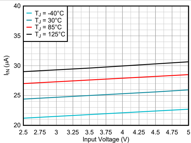
图 6-2. 静态电流
