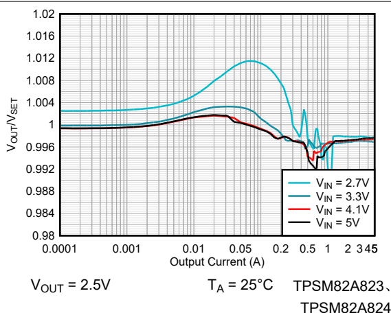
图 8-16. VOUT 精度
