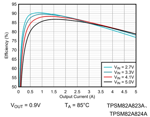
图 8-35. 效率
