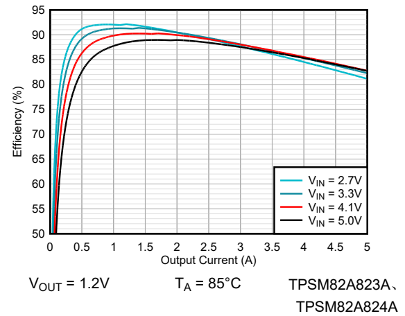
图 8-33. 效率
