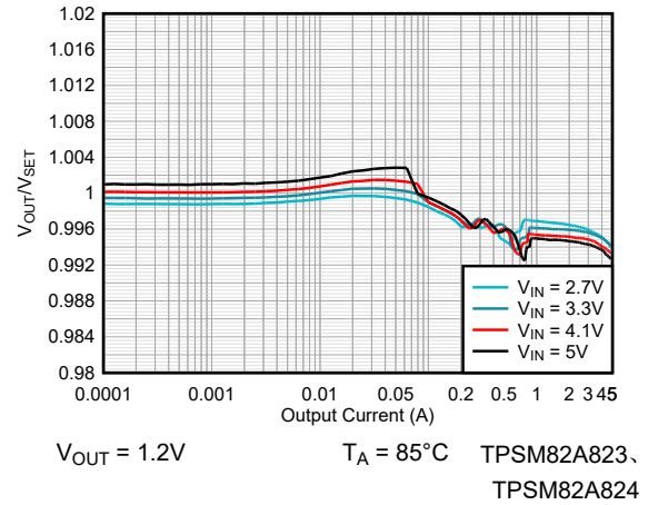
图 8-21. VOUT 精度
