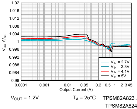
图 8-20. VOUT 精度
