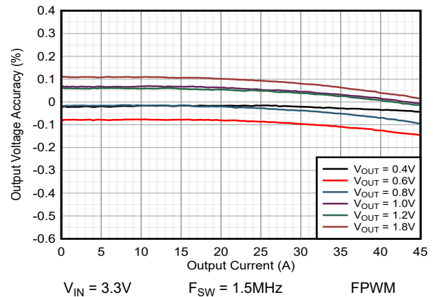
图 9-44. 负载调整率
