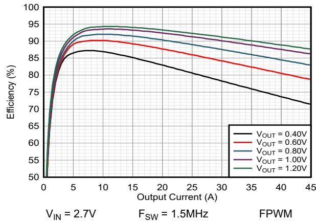
图 9-41. 效率
