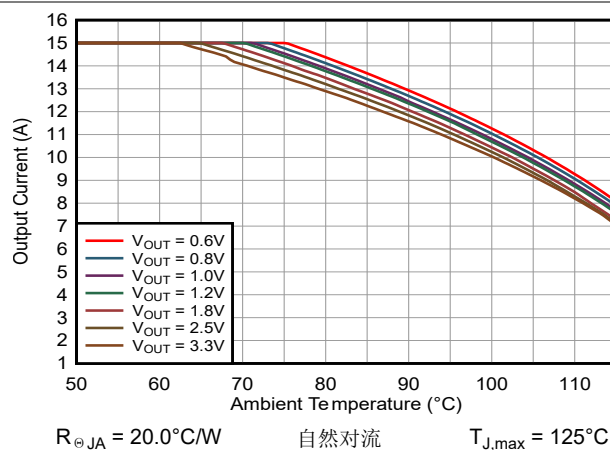
图 9-39. TPSM8287A15BBM 安全工作区, V_{IN} = 5.0\text{V}
