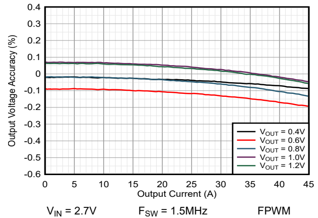
图 9-42. 负载调整率
