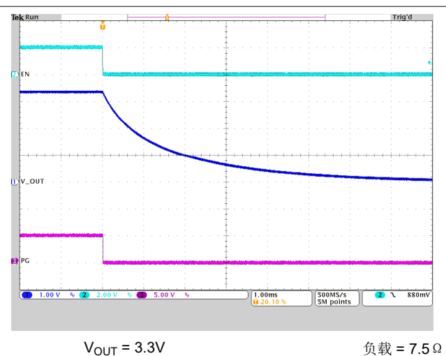
图 9-31. 通过 EN 引脚关断 ( 禁用放电 )
