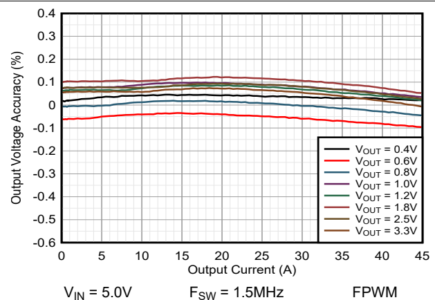
图 9-46. 负载调整率
