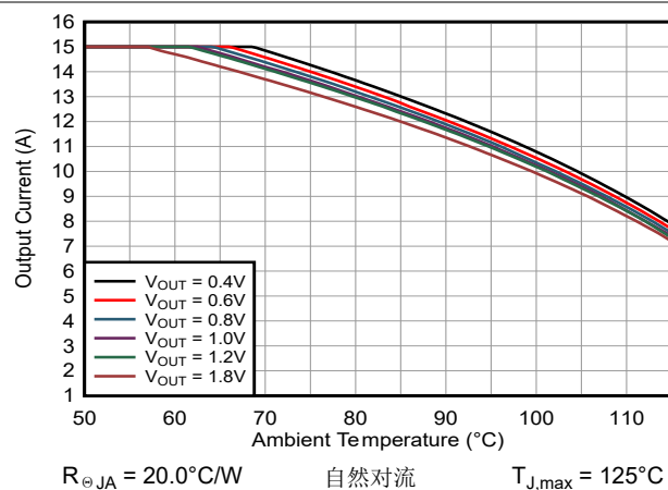
图 9-38. TPSM8287A15BBM 安全工作区, V_{IN} = 3.3\text{V}
