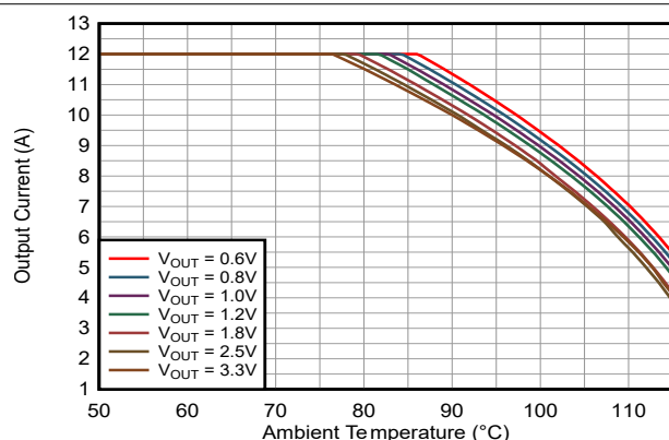
图 9-33. TPSM8287A12BAM 安全工作区, V_{IN} = 5.0\text{V}
