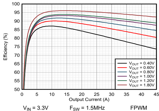
图 9-43. 效率
