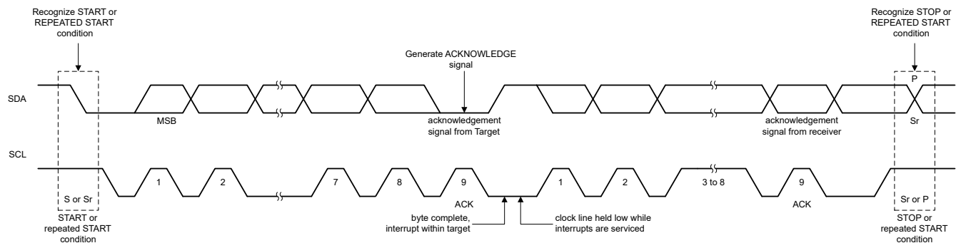
图 7-26. Bus Protocol
