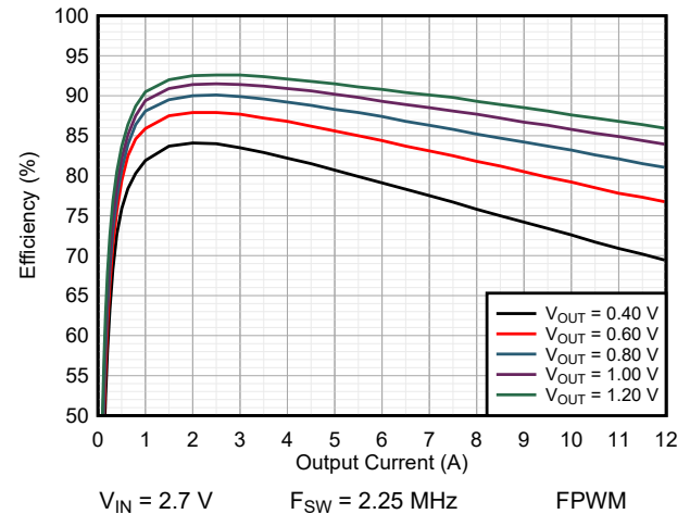
图 9-9. Efficiency TPSM8287A12BBS
