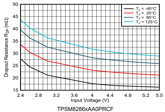
图 6-6. Dropout Resistance R_{DP}
