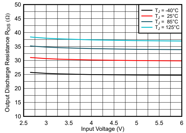
图 6-4. Discharge Resistance
