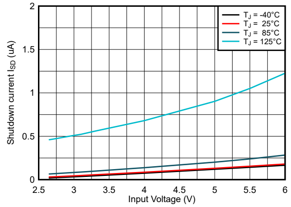
图 6-2. Shutdown Current
