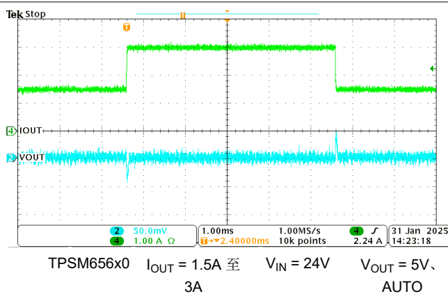
图 8-7. 负载瞬态 (50% 至 100%)
