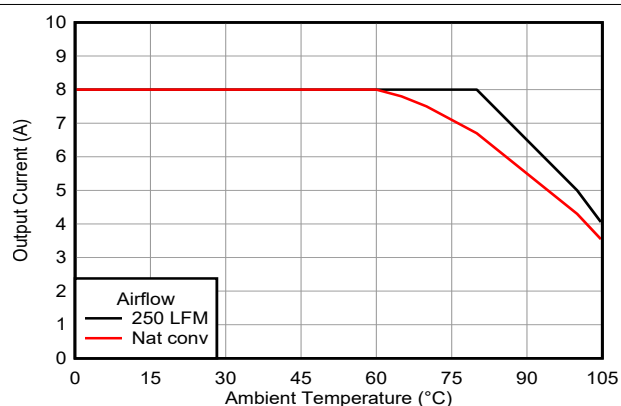
图 6-12. EVM 热性能 ( V_{IN} = 24V , V_{OUT} = 3.3V , F_{SW} = 700kHz )
