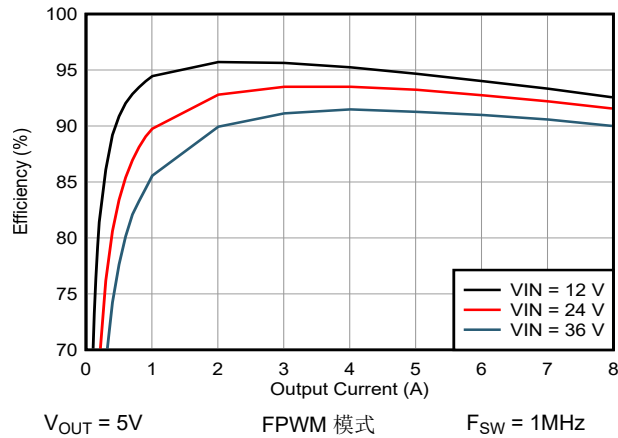
图 8-2. V_{OUT} = 5V 时的效率
