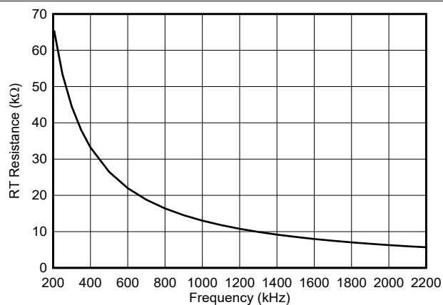
图 6-8. 通过 RT 电阻设置的开关频率
