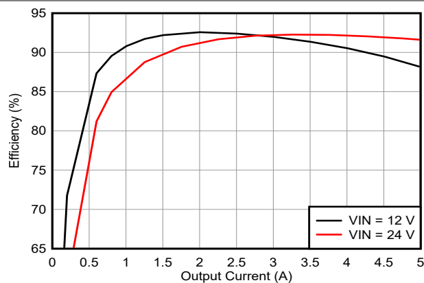
图 8-16. 效率, V_{OUT} = -12V , FPWM 模式
