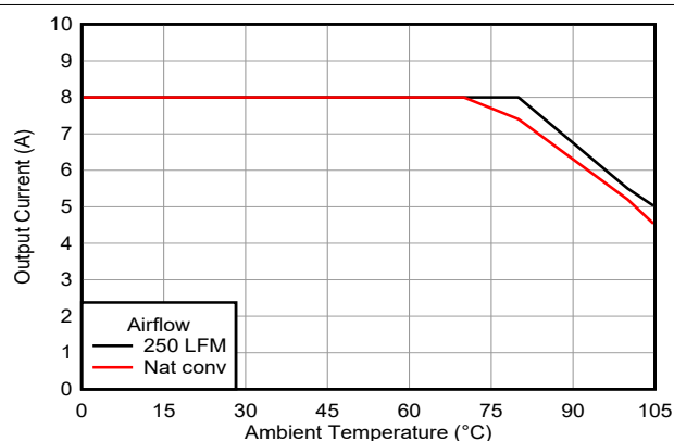
图 6-11. EVM 热性能 ( V_{IN} = 12V , V_{OUT} = 3.3V , F_{SW} = 700kHz )
