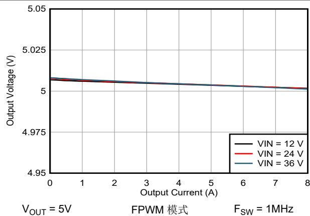
图 8-4. V_{OUT} = 5V 时的负载调节
