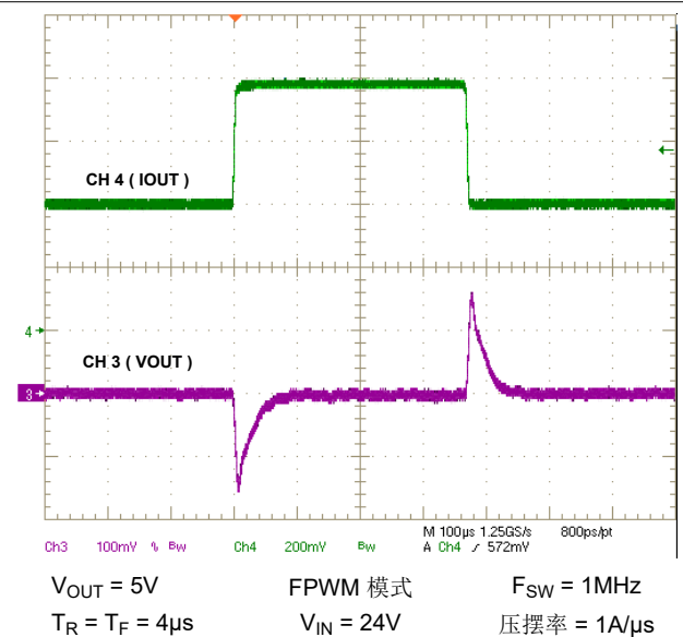
图 8-7. 瞬态负载，在 1A/\mu s 下为 4A 至 8A
