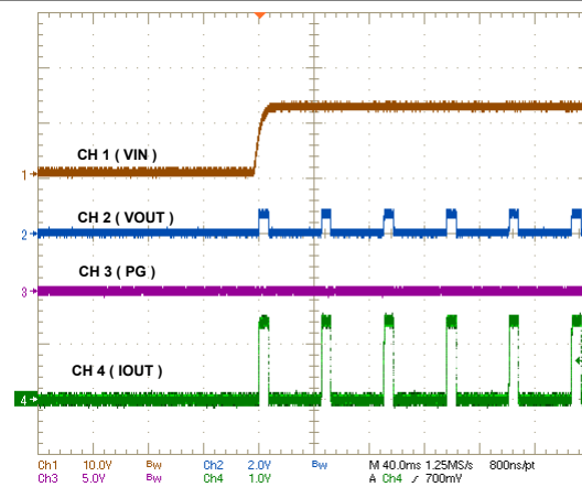
图 8-9. 启动至短路
