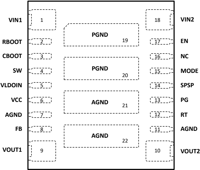
图 5-1. 22 引脚 B3QFN RDF 封装（顶视图）
