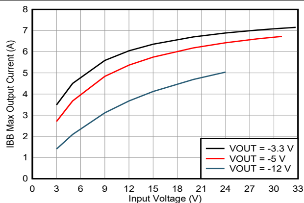
图 8-15. IBB 最大输出电流
