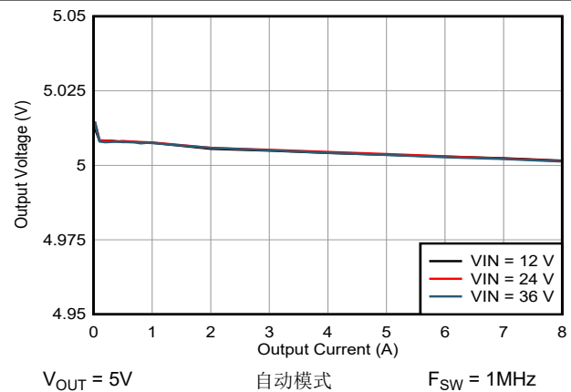
图 8-5. V_{OUT} = 5V 时的负载调节
