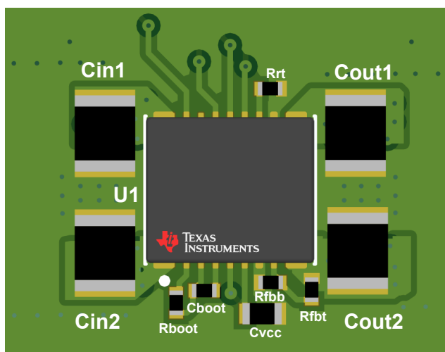
图 8-17. 典型布局
