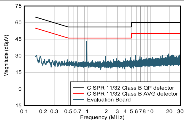
图 8-11. CISPR 11/32 B 类传导发射: V_{IN} = 24V , SPSP 关闭
