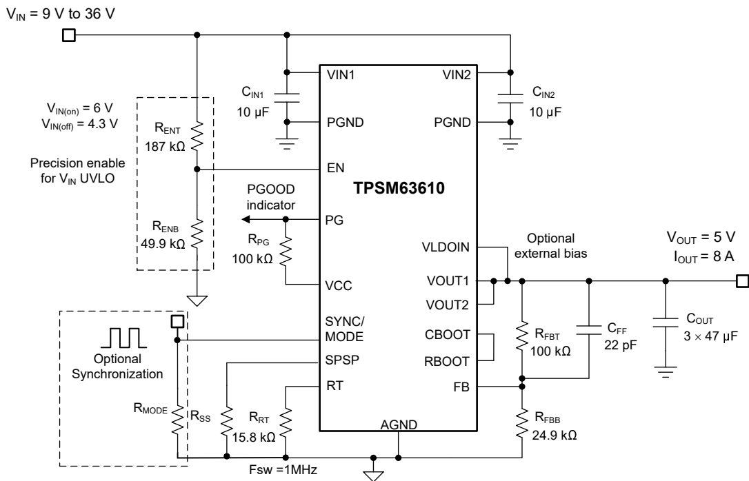
图 8-1. 电路原理图
