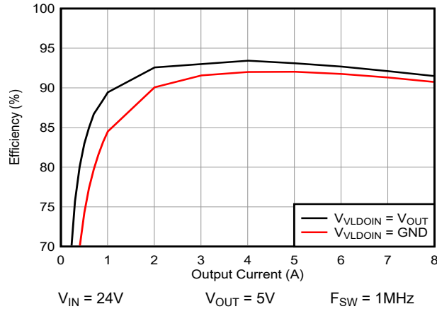
图 7-6. 通过外部偏置提高效率
