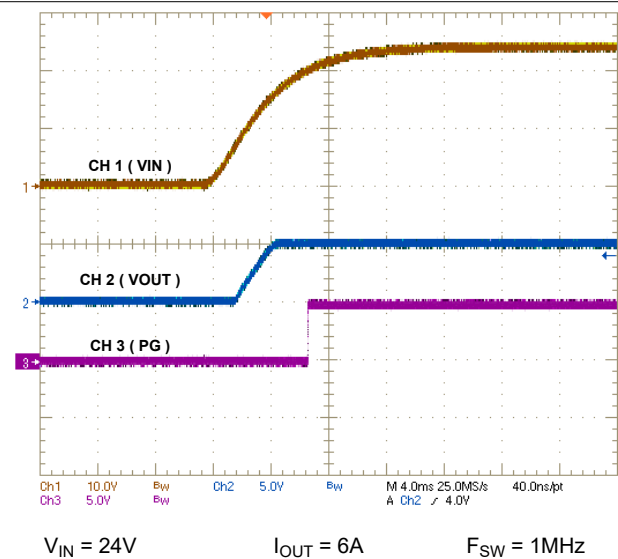
图 8-6. 启动
