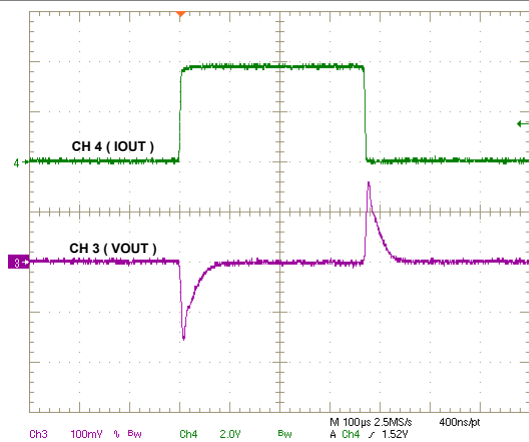
图 8-8. 瞬态负载, 在 1A/\mu s 下为 0A 至 4A
