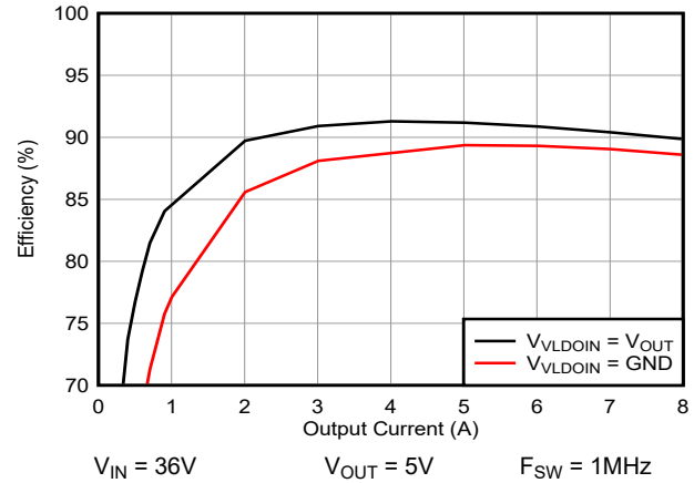
图 7-7. 通过外部偏置提高效率
