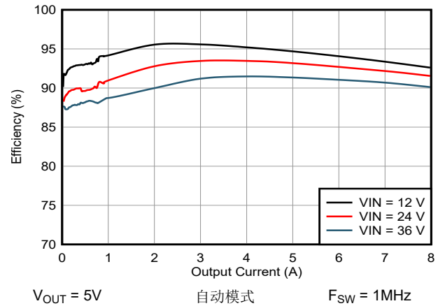
图 8-3. V_{OUT} = 5V 时的效率
