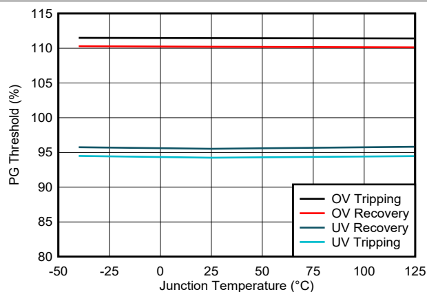
图 6-7. 电源正常 (PG) 阈值
