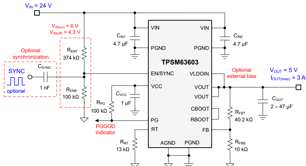
图 8-1. 电路原理图
