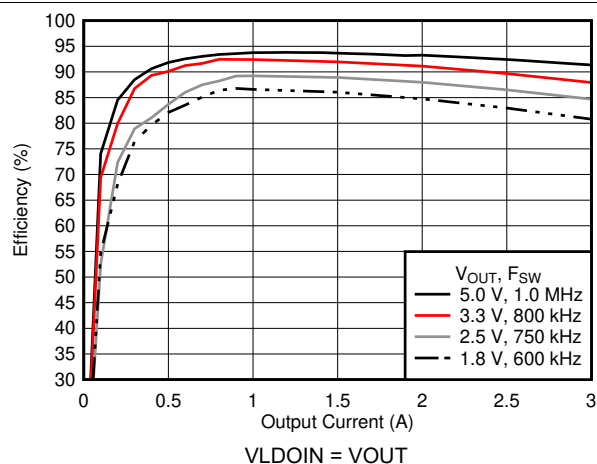
图 6-7. 效率
