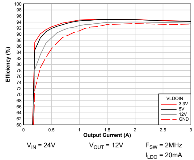
图 7-9. 通过 VLDOIN 实现的效率提升 ( V_{OUT} = 12V )
