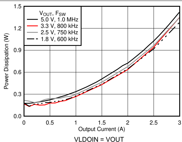
图 6-8. 功率耗散
