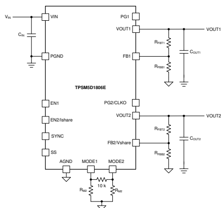
双路输出简化版原理图
