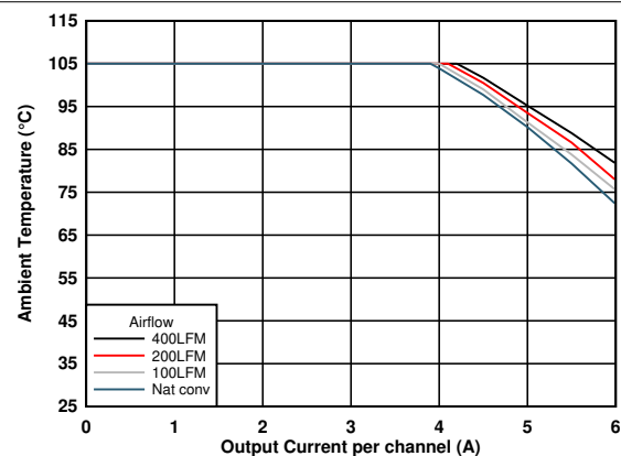
图 6-10. Maximum Output Current
