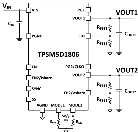
双路输出简化版原理图
