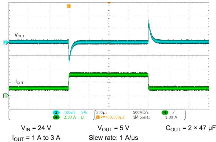
图 8-4. Transient Response
