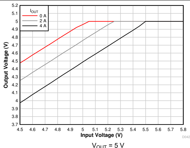
图 7-9. Voltage Dropout
