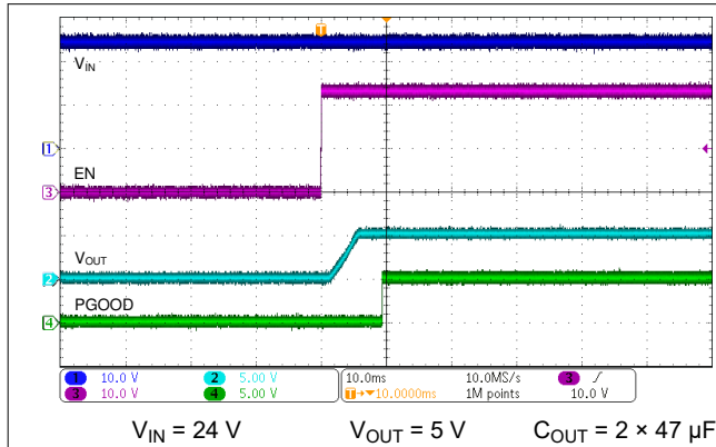
图 8-2. Enable Turn-ON
