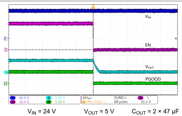
图 8-3. Enable Turn-OFF
