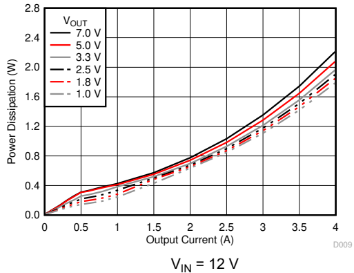
图 6-9. Power Dissipation versus Output Current
