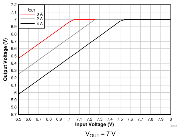
图 7-11. Voltage Dropout
