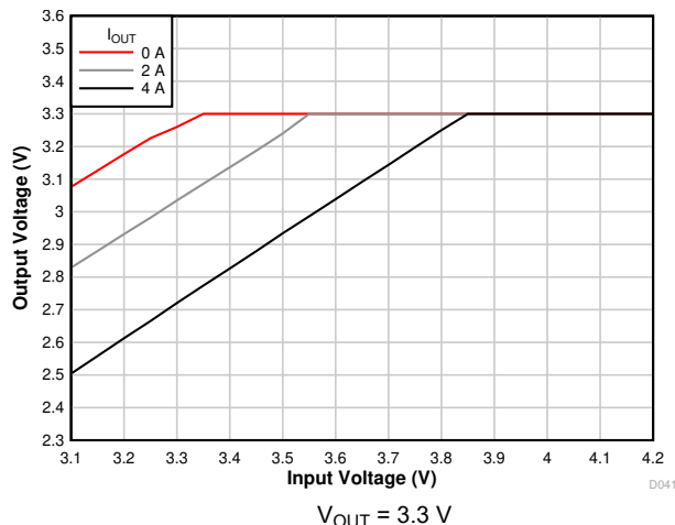
图 7-7. Voltage Dropout
