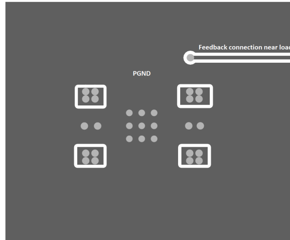
图 10-3. Typical PGND Layer
