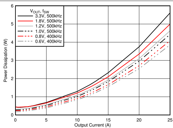
图 6-9. Power Dissipation vs Output Current
