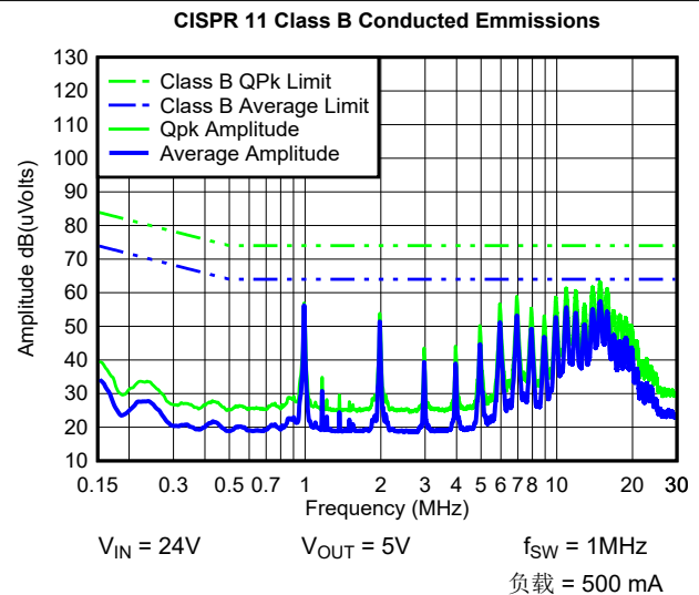
图 8-12. 典型 CISPR 11 B 类传导 EMI 150kHz 至 30MHz, 不带 EMI 滤波器 (标准 EVM 布局和 BOM)
