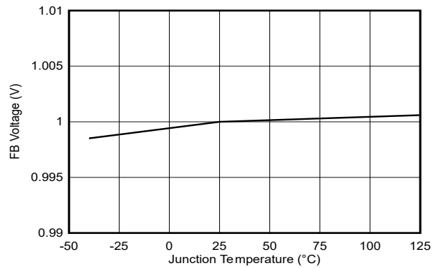
图 6-2. 反馈电压
