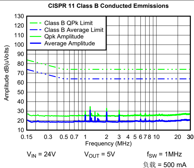
图 8-11. 典型 CISPR 11 B 类传导 EMI 150kHz 至 30MHz, 带 EMI 滤波器 (标准 EVM 布局和 BOM)
