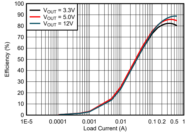
图 6-10. FPWM 模式下的效率
