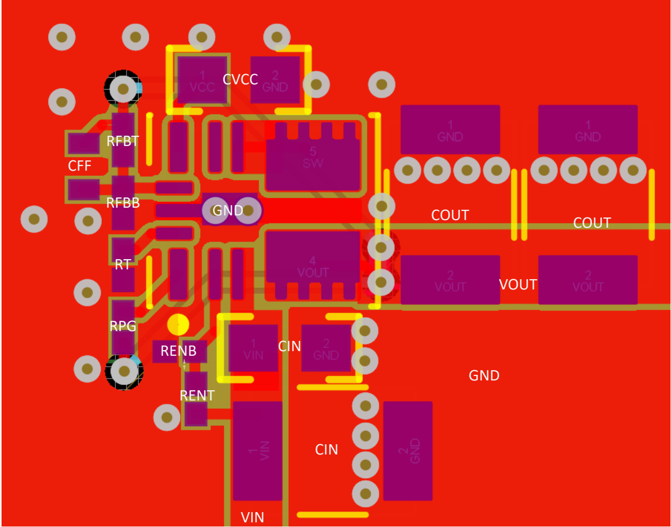
图 8-15. 布局示例
