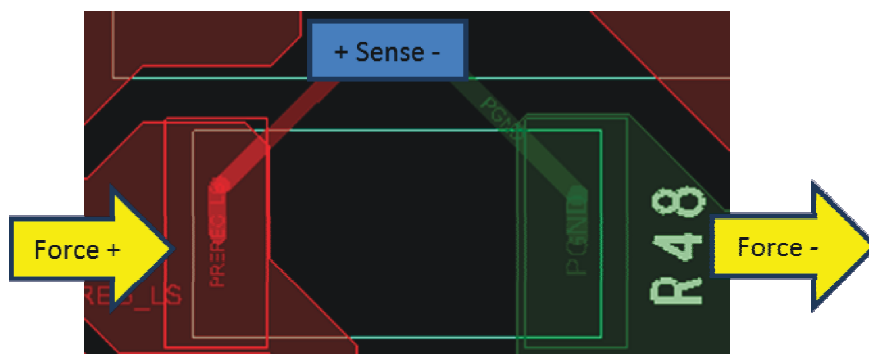
图 9-3. Kelvin Sensing Layout
