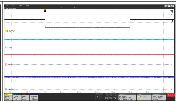
图 6-14. Transient Undervoltage
