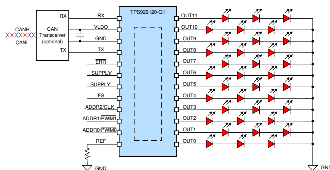
典型应用图
