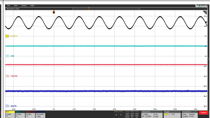
图 6-16. Jump Start
