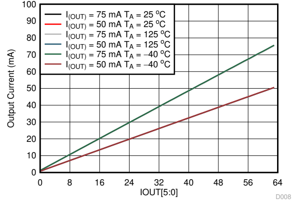
图 6-8. Output DC Current vs IOUT[5:0]
