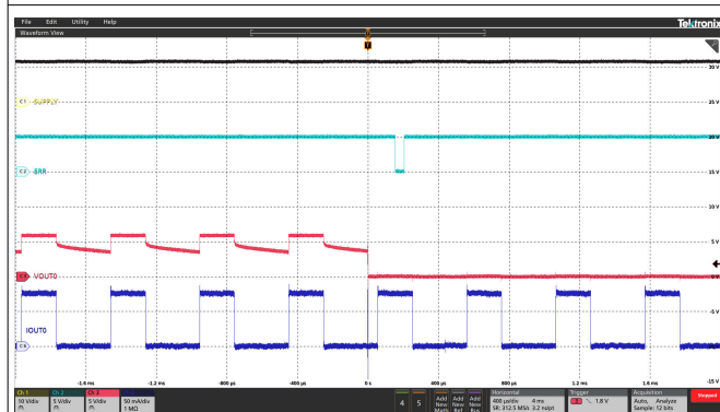
图 6-21. LDO Output Load Transient
