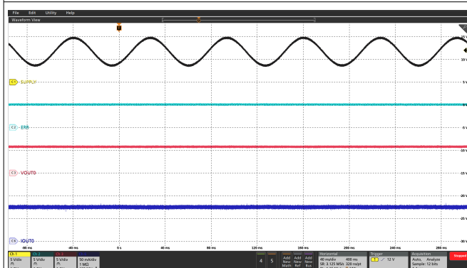
图 6-15. Transient Overvoltage
