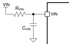
图 8-3. VIN Filter
