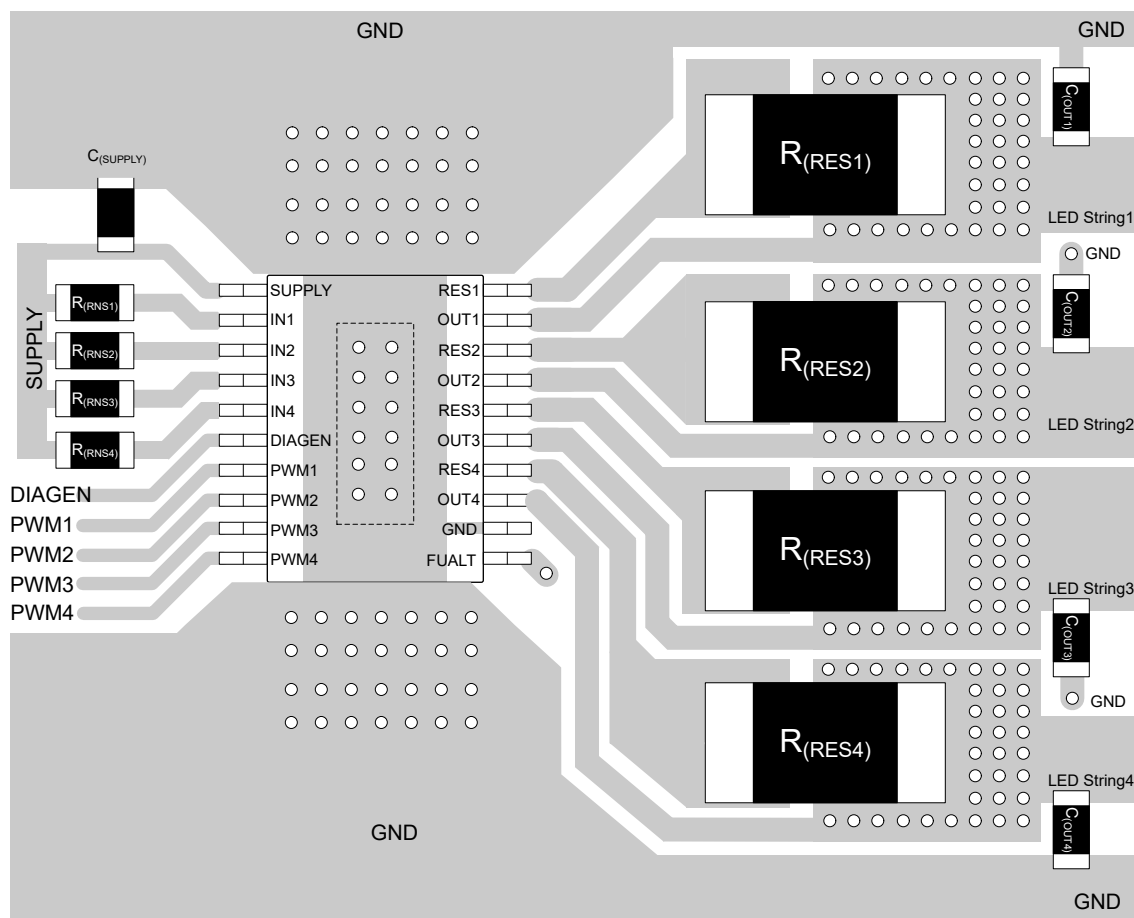
图 10-1. TPS92624-Q1 Example Layout Diagram
