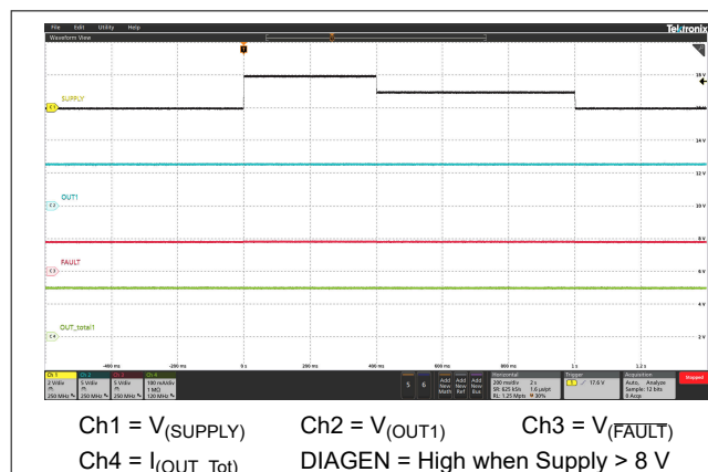
图 6-19. Transient Overvoltage
