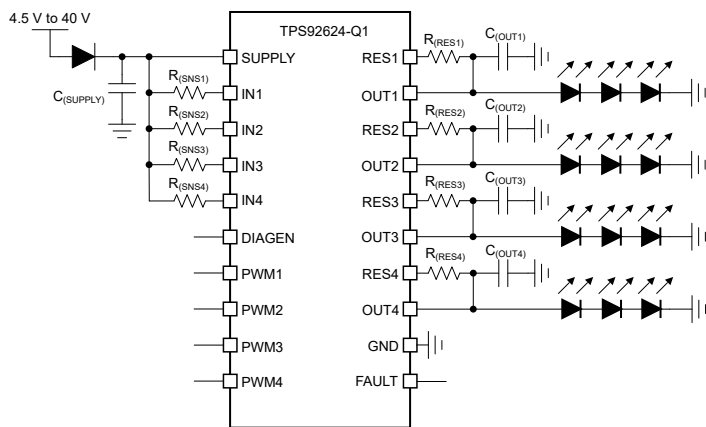
典型应用图
