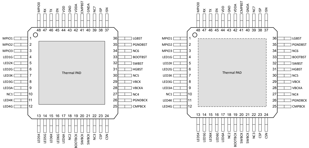
图 4-1. PKD 封装 48 引脚 HTQFP (顶部外露焊盘) 顶视图
