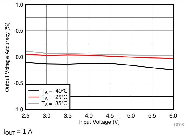
图 17. Line Regulation
