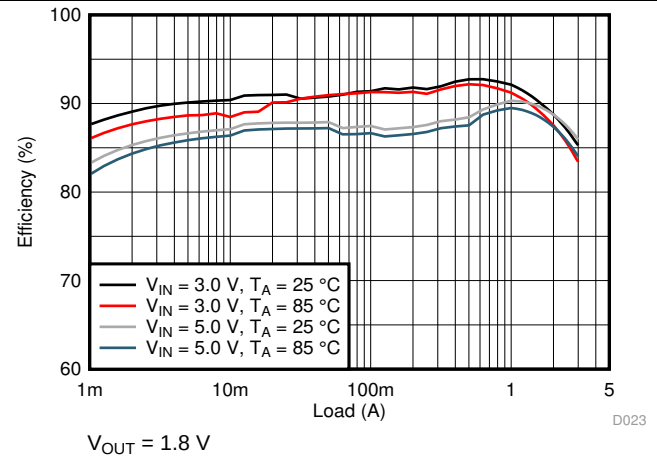
图 9. Efficiency
