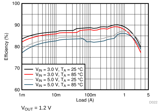
图 7. Efficiency
