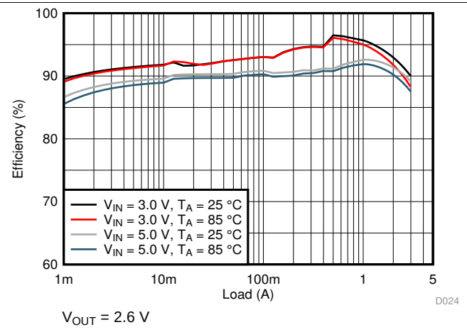
图 11. Efficiency
