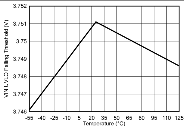
图 6-5. VIN UVLO 下降阈值与温度间的关系
