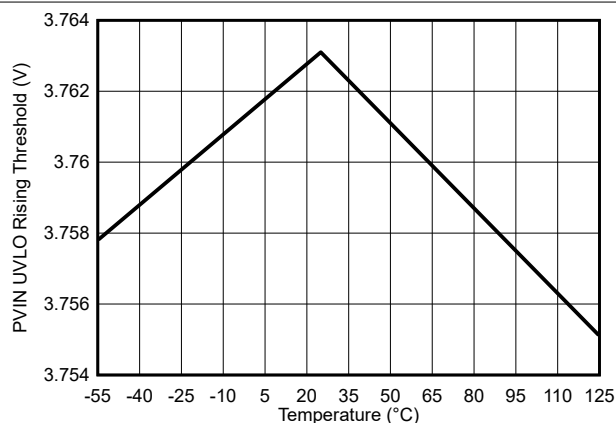
图 6-6. PVIN UVLO 上升阈值与温度间的关系
