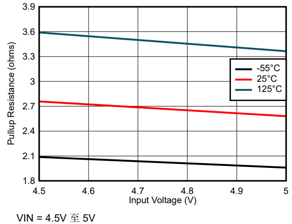
图 6-24. 上拉电阻与输入电压间的关系
