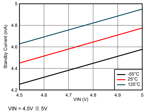
图 6-32. 待机电流与输入电压间的关系
