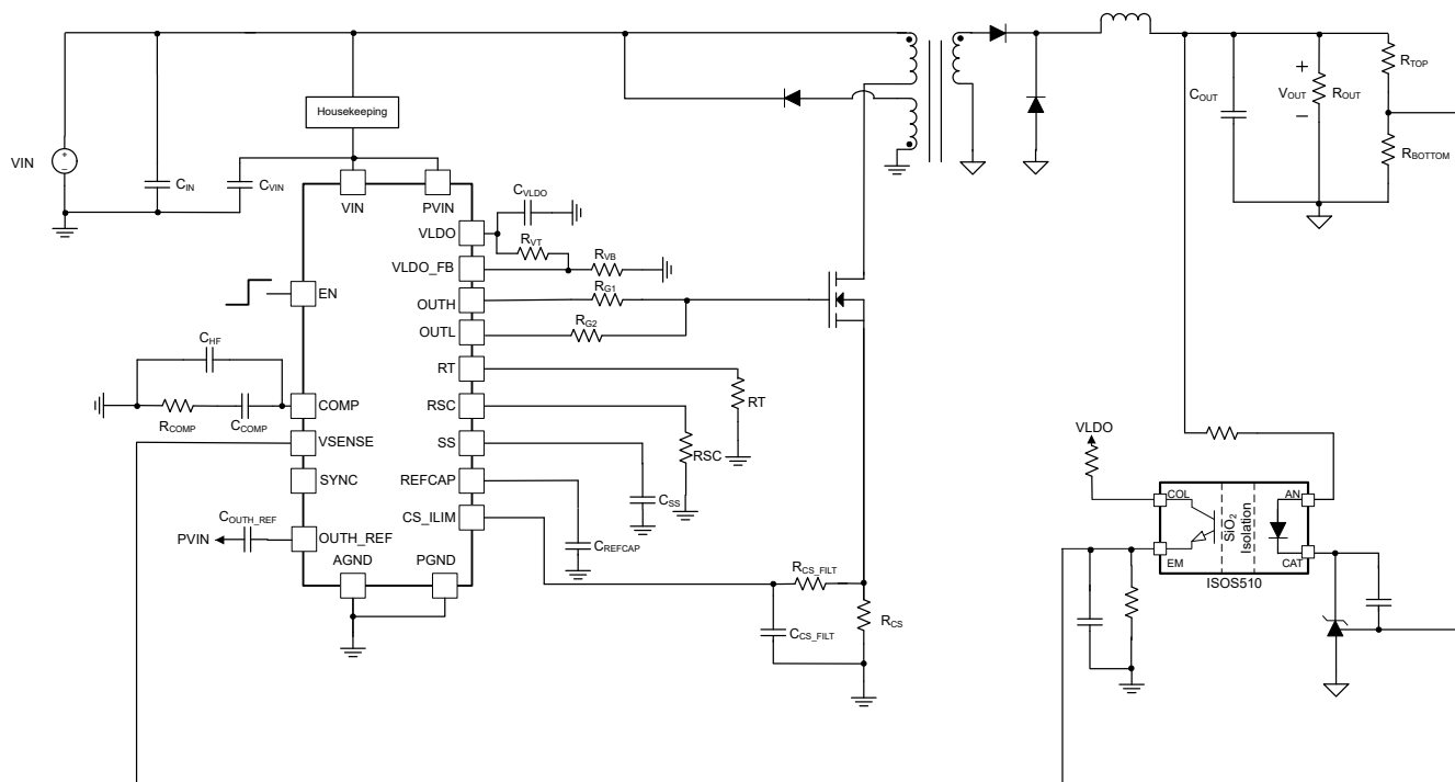
图 8-6. 使用 TPS7H502x 控制器和 ISOS510 实现反馈的正激式转换器
