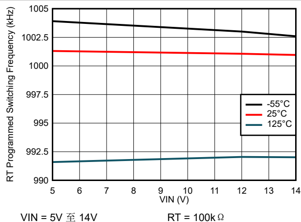
图 6-19. 开关频率与输入电压间的关系
