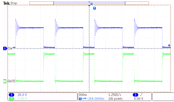
图 8-4. 栅极和开关节点信号
