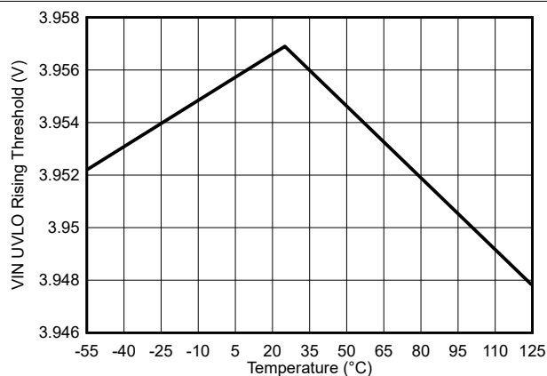
图 6-4. VIN UVLO 上升阈值与温度间的关系
