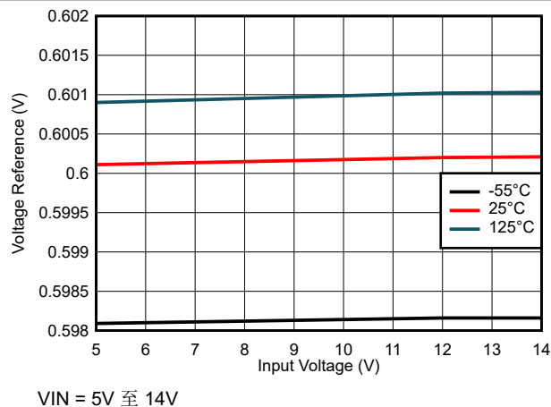
图 6-21. 内部电压基准与输入电压间的关系
