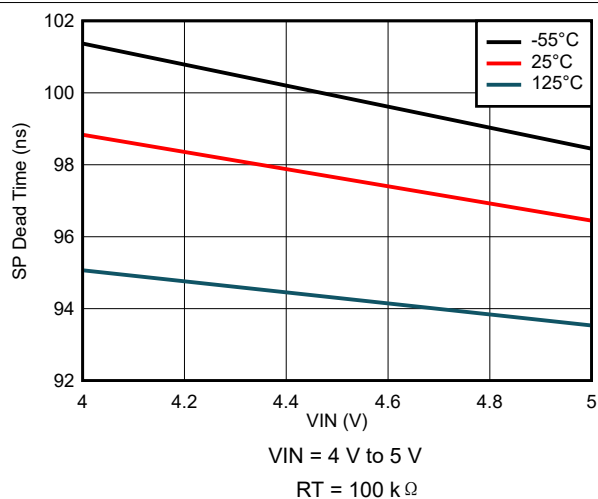
图 7-53. SP Dead Time Variation
