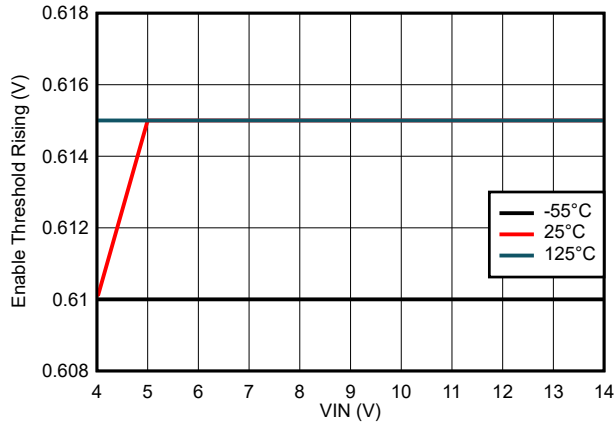
图 8-7. Enable Threshold Rising Variation
