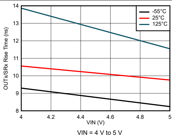
图 8-57. Output Rise Time Variation
