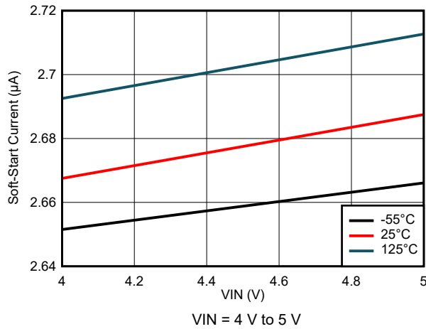
图 8-9. Soft-Start Current Variation
