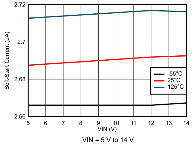
图 8-10. Soft-Start Current Variation
