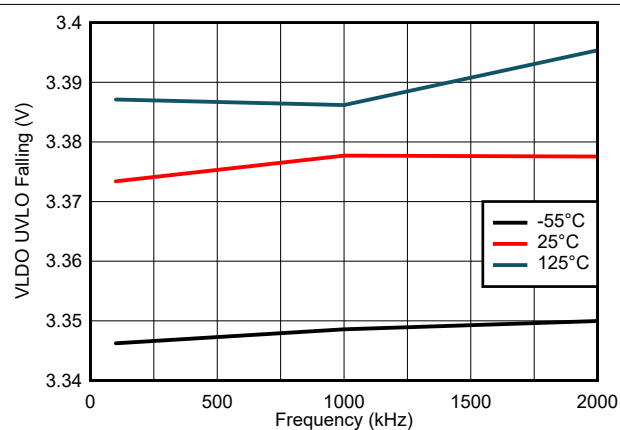
图 8-6. VLDO UVLO Falling Variation
