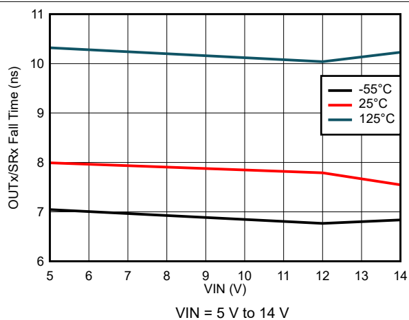
图 8-60. Output Fall Time Variation
