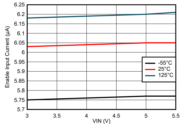
图 6-6. Enable Input Current Variation
