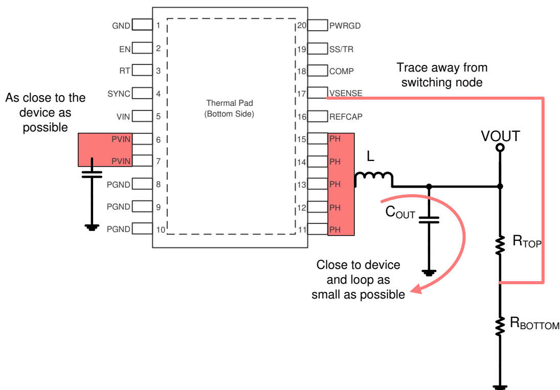
图 10-1. PCB Layout Example
