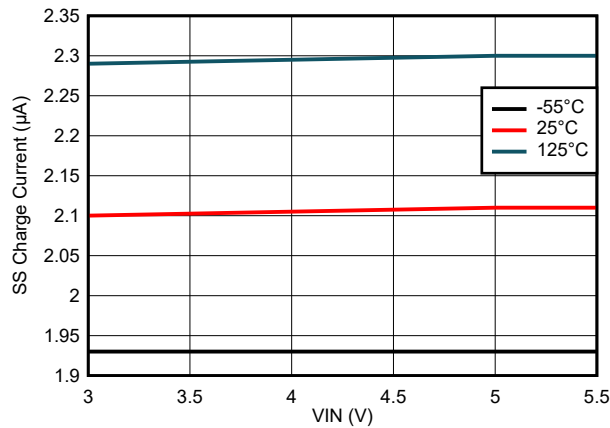
图 6-9. SS Charge Current Variation
