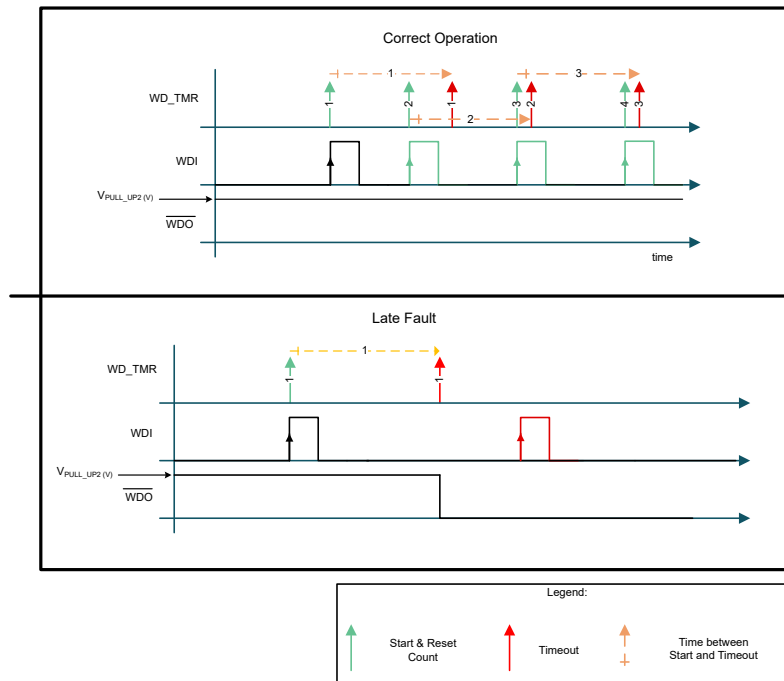
图 8-21. 看门狗时序图
