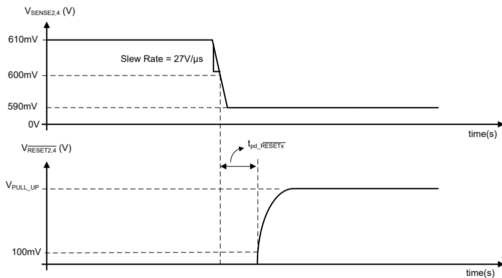
图 7-6. TPS7H31x4 (漏极开路) 的 \overline{\text{RESET2}} 和 \overline{\text{RESET4}} 传播延迟 ( t_{\text{pd\_RESETx}} ) 时间测量
