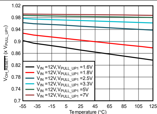
图 6-26. I_{LOAD} = 10mA 时, 不同 V_{PULL\_UP1} 下作为 V_{PULL\_UP1} 百分比的 RESET1 VOH 电压与温度间的关系
