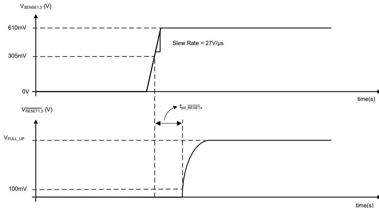
图 7-5. TPS7H31x4 (漏极开路) 的 \overline{\text{RESET1}} 和 \overline{\text{RESET3}} 传播延迟 ( t_{\text{pd\_RESETx}} ) 时间测量
