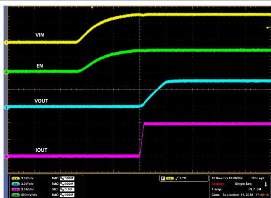
图 9-4. TPS7H2201SP 的上电行为
