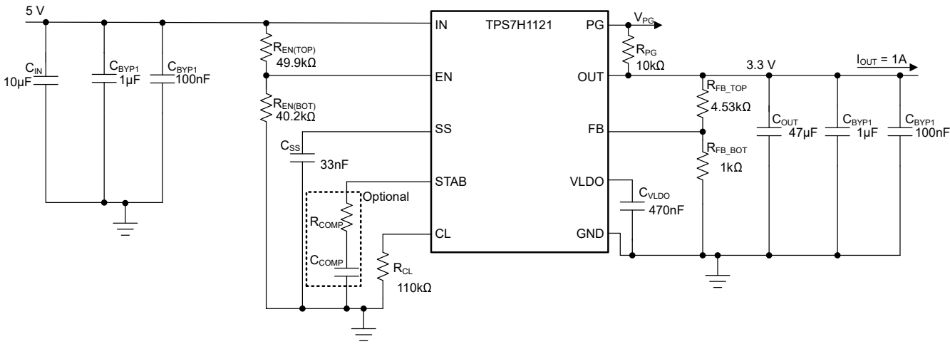
图 9-1. 应用原理图
