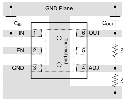
图 7-12. TPS7E82 ( DRV 封装 ) 的布局示例
