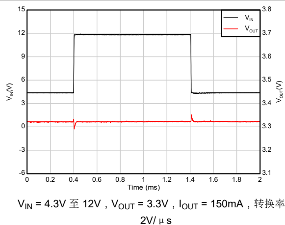
图 5-30. 线路瞬态
