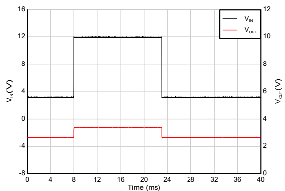
图 5-32. 线路瞬态
