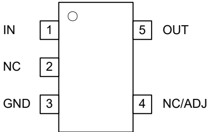
图 4-4. DBV 封装, [A 版本、无 EN] (固定/ADJ)，5 引脚 SOT-23 (顶视图)
