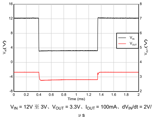
图 5-47. 压降恢复 (12V 至 3V)
