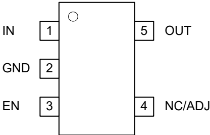
图 4-3. DBV 封装 (固定/ADJ)，5 引脚 SOT-23 (顶视图)
