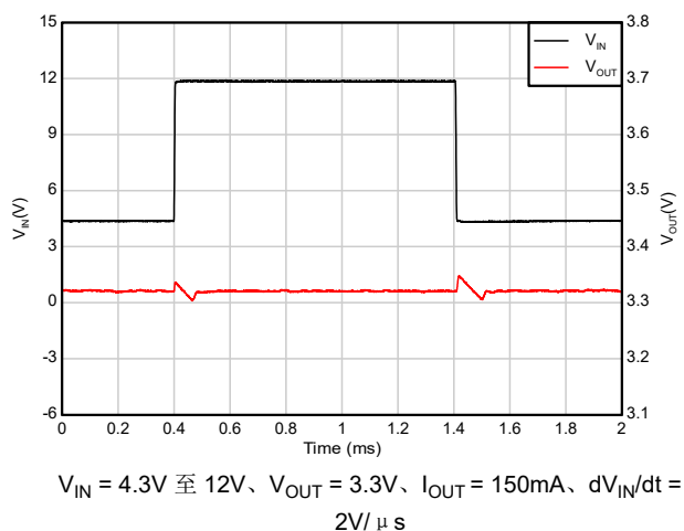
图 7-12. 线路瞬态 (4.3V 至 12V)
