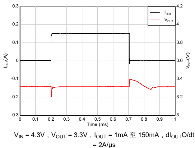
图 7-14. 负载瞬态 (1mA 至 150mA)
