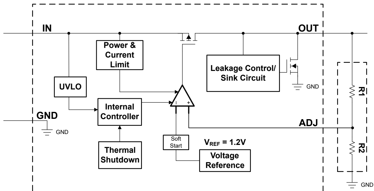
图 6-3. 功能方框图：可调节版本 (无 EN 功能)
