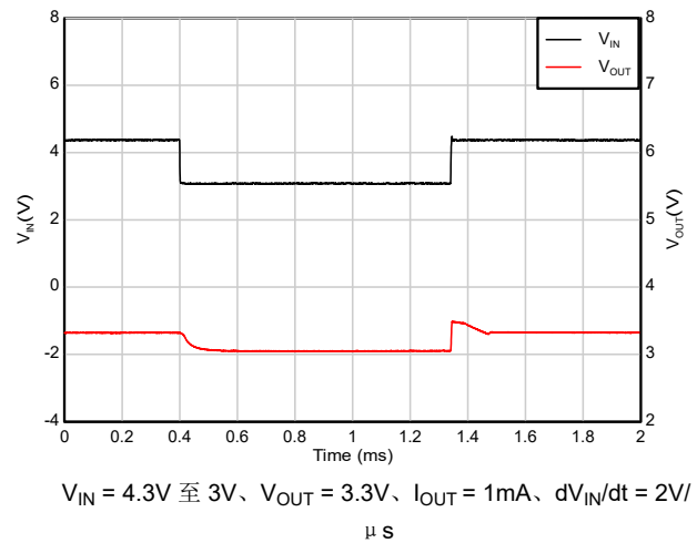
图 5-44. 压降恢复 (4.3V 至 3V)
