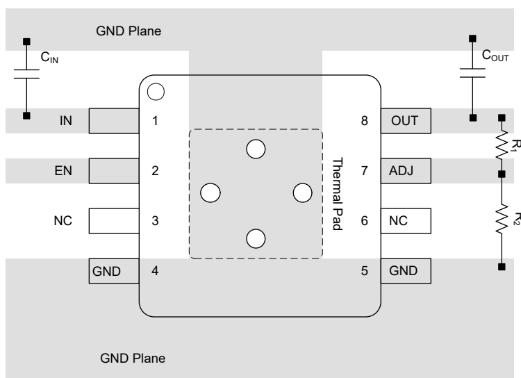
图 7-19. DGN 封装的布局示例
