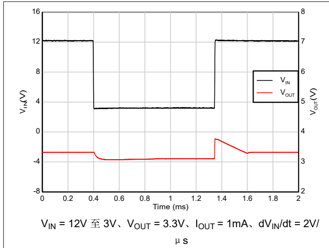
图 7-15. 压降恢复 (12V 至 3V)
