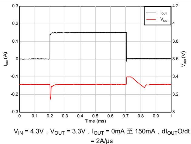
图 7-13. 负载瞬态 (0mA 至 150mA)
