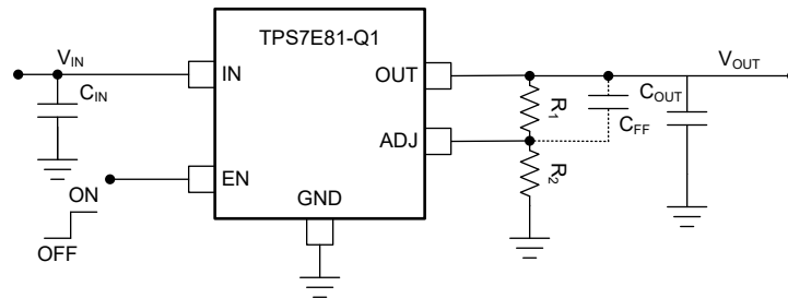
图 7-6. 可调节 LDO 稳压器编程
