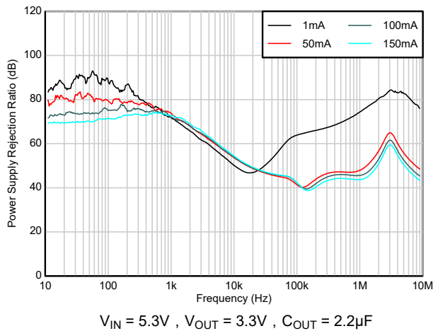
图 5-19. PSRR 与 I_{OUT} 间的关系
