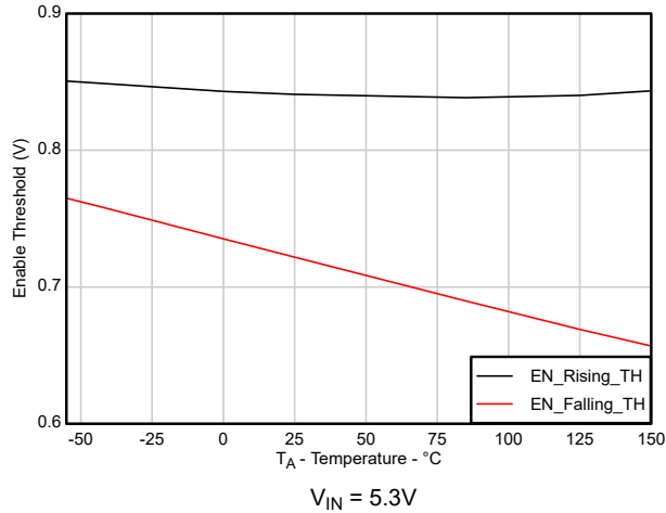
图 5-13. EN 阈值 V_{IH(EN)}/V_{IL(EN)} 与温度间的关系
