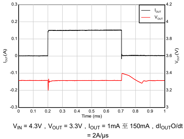
图 5-43. 负载瞬态 (1mA 至 150mA)
