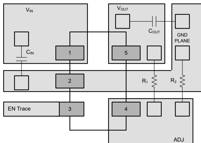
图 7-20. DBV 封装的布局示例
