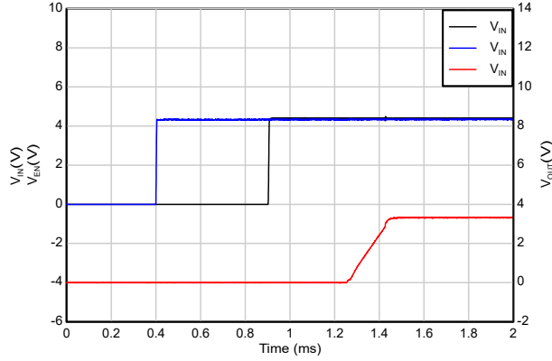
图 5-37. 时序启动 ( V_{IN} 在 V_{EN} 之后)
