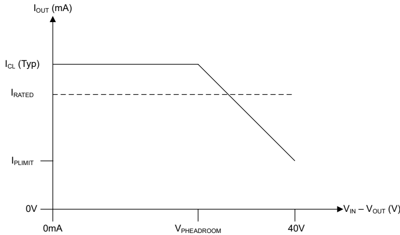
图 6-6. 功率限制
