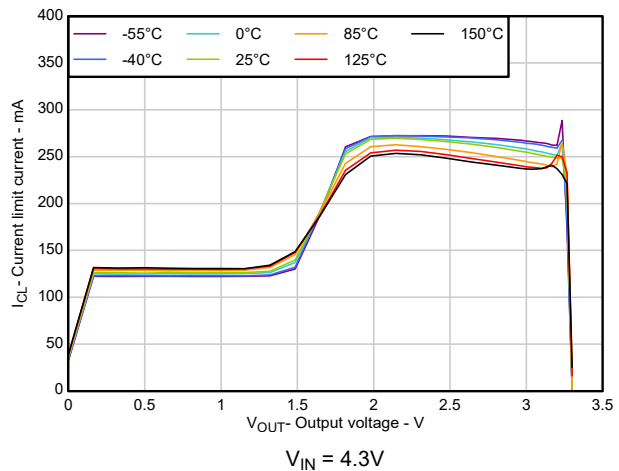
图 5-12. 折返电流限值 I_{CL} 与温度间的关系
