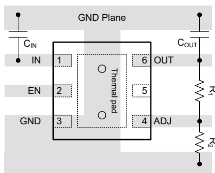
图 7-22. DRV 封装的布局示例
