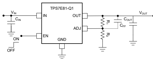
图 3-1. 典型应用
