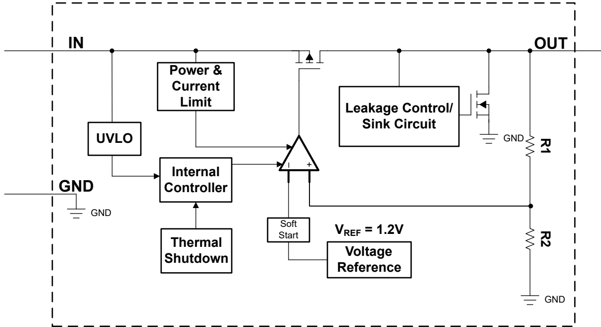
图 6-4. 功能方框图：固定版本（无 EN 功能）
