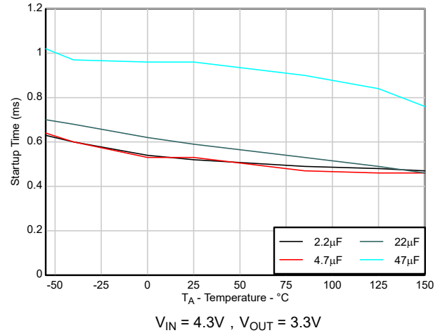
图 5-18. 启动时间与 C_{OUT} 间的关系
