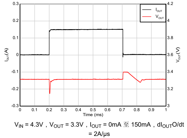
图 5-42. 负载瞬态 (0mA 至 150mA)
