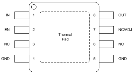
图 4-5. DGN 封装 (固定/ADJ)，8-引脚 HVSSOP (顶视图)
