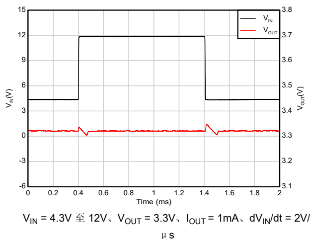
图 7-11. 线路瞬态 (4.3V 至 12V)
