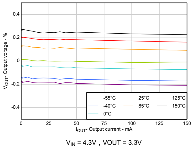
图 2-1. V_{OUT} 精度与 I_{OUT} 间的关系
