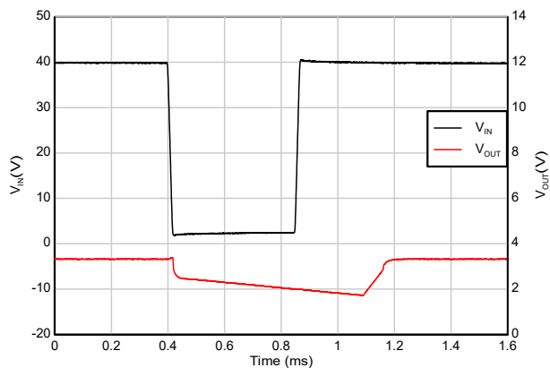
图 5-50. 欠压恢复 (40V 至 2V)
