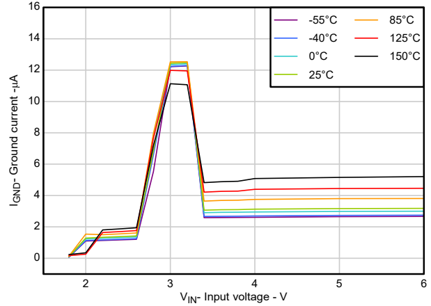
图 5-8. I_{GND} 与 V_{IN} 间的关系
