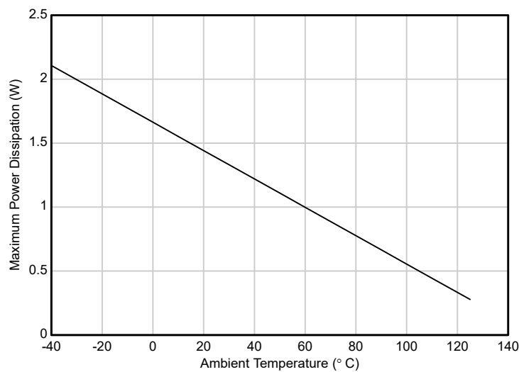
图 7-3. TPS7E81-Q1 (DRV) 允许的功率耗散
