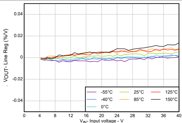
图 5-4. 线路调整率
