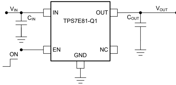
图 7-5. 典型应用电路 (固定电压版本)
