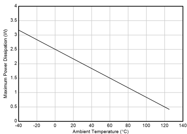
图 7-4. TPS7E81-Q1 (DGN) 允许的功率耗散
