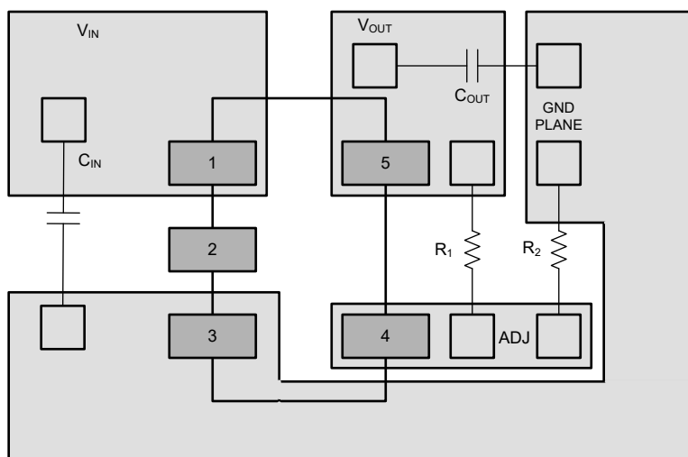
图 7-21. DBV-A (无 EN 功能) 封装的布局示例
