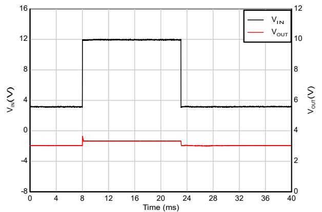
图 5-46. 压降恢复 (12V 至 3V)
