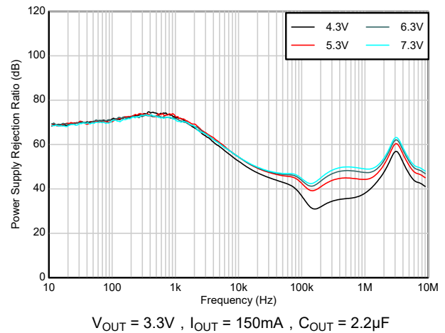
图 5-20. PSRR 与 V_{IN} 间的关系
