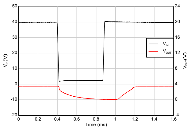
图 5-49. 冷启动恢复
