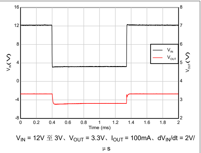
图 7-16. 压降恢复 (12V 至 3V)
