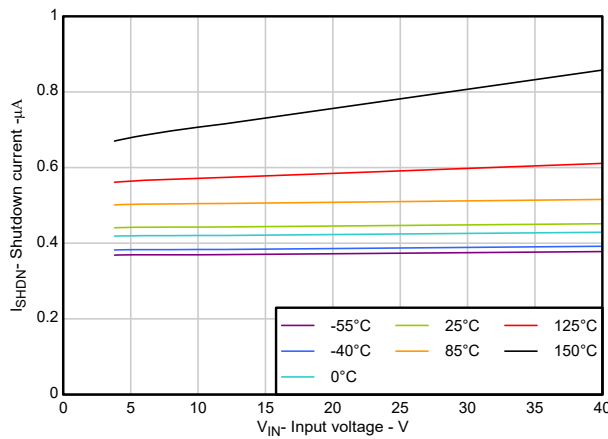
图 5-11. I_{GSHDN} 与 V_{IN} 间的关系
