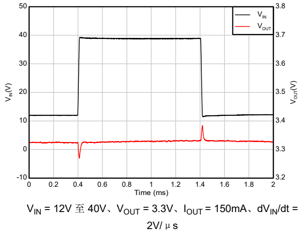
图 5-41. 线路瞬态 (12V 至 40V)
