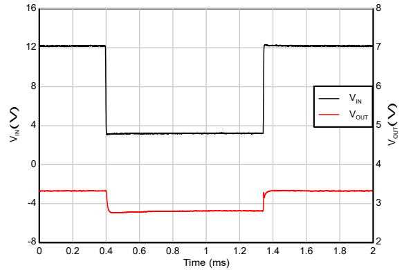
图 5-38. 压降恢复
