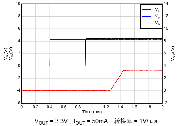
图 7-9. 时序启动 ( IN 在 EN 之后 )
