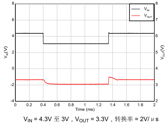
图 5-37. 压降恢复
