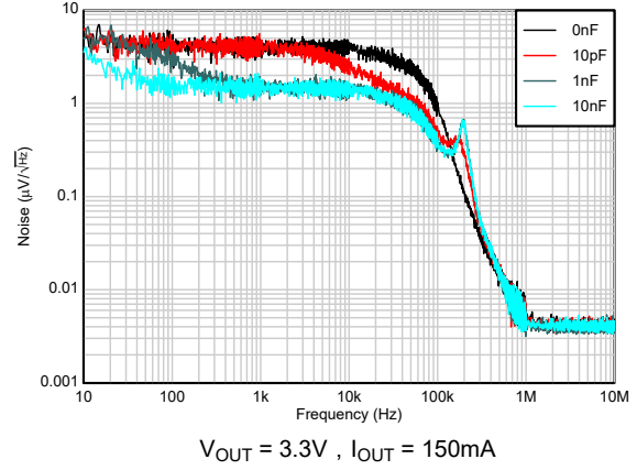
图 5-26. 输出噪声与频率和 C_{FF} 之间的关系
