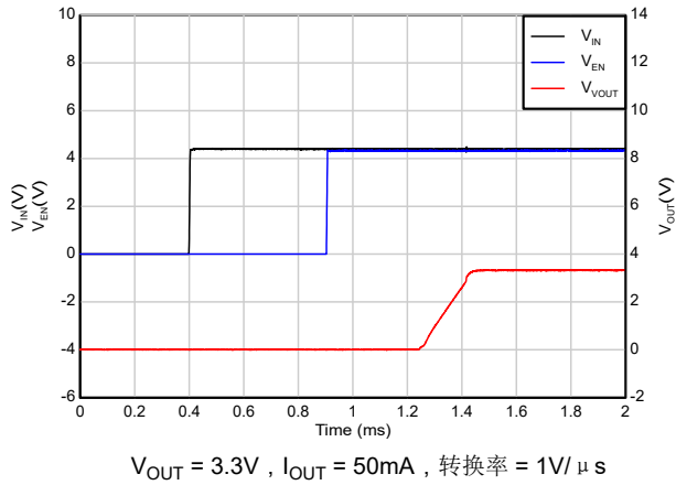
图 7-8. 时序启动 ( EN 在 IN 之后 )
