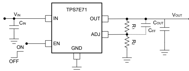
典型应用
