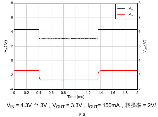
图 5-38. 压降恢复
