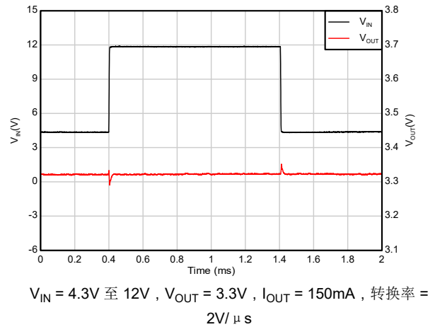
图 5-30. 线路瞬态
