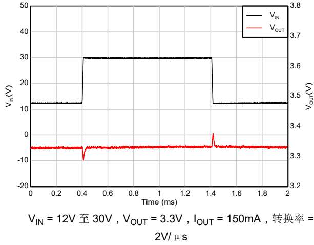
图 7-6. 线路瞬态
