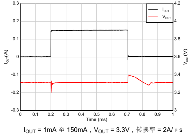
图 7-7. 负载瞬态
