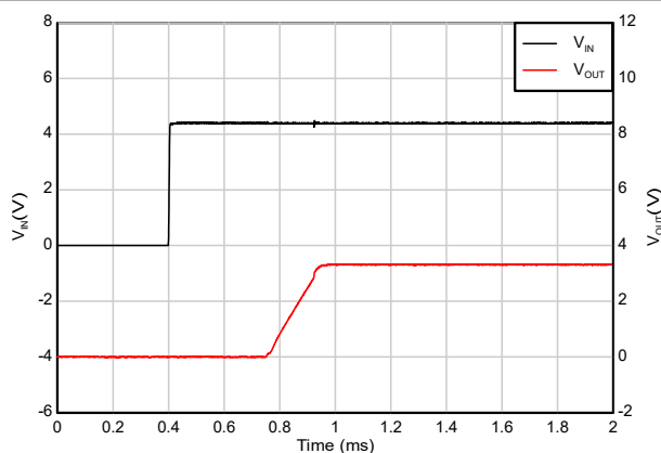
图 7-10. IN 与 EN 引脚短接启动
