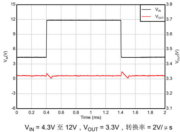
图 5-29. 线路瞬态
