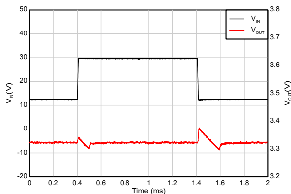
图 5-31. 线路瞬态
