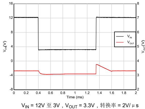
图 5-39. 压降恢复
