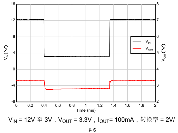
图 5-40. 压降恢复
