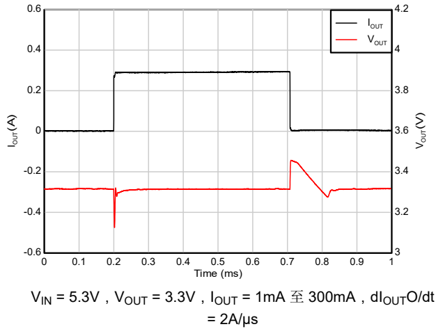
图 7-11. 负载瞬态 (1mA 至 300mA)
