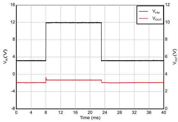
图 5-48. 压降恢复 (12V 至 3V)
