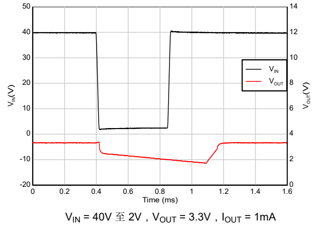
图 5-52. 欠压恢复 (40V 至 2V)
