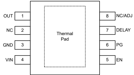
图 4-4. DDA 封装 (固定/ADJ), 8-引脚 HSOIC (顶视图)
