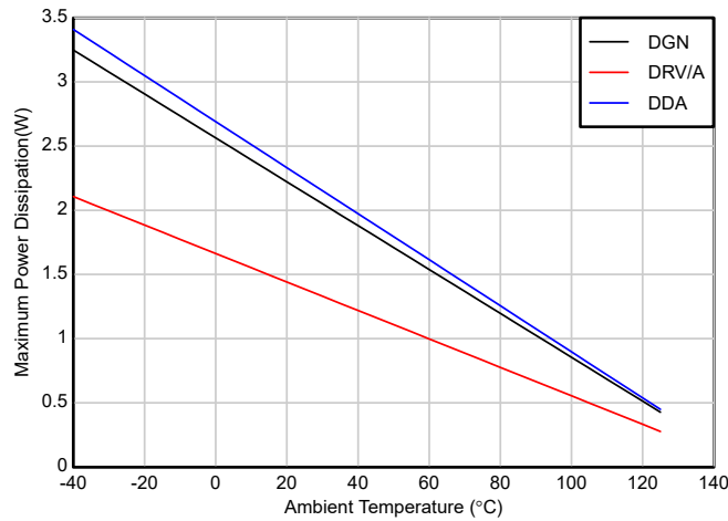
图 7-2. TPS7E67-Q1 允许的功率耗散
