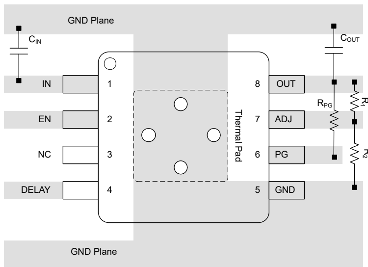
图 7-16. TPS7E67-Q1 DGN 封装的布局示例
