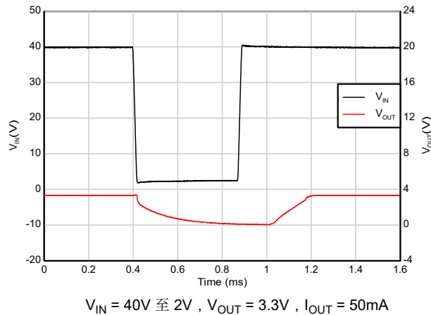
图 5-53. 欠压恢复 (40V 至 2V)
