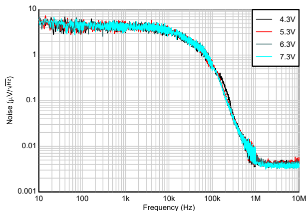
图 5-27. 噪声与 V_{IN} 间的关系
