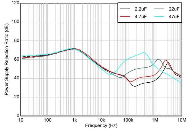
图 5-24. PSRR 与 C_{OUT} 间的关系
