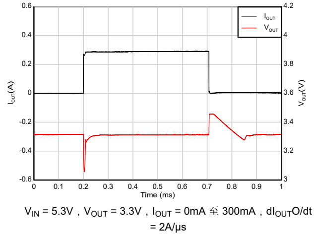
图 7-10. 负载瞬态 (0mA 至 300mA)
