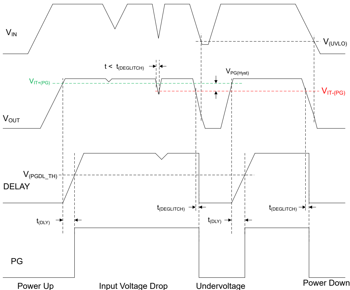
图 6-3. 典型的电源正常时序图
