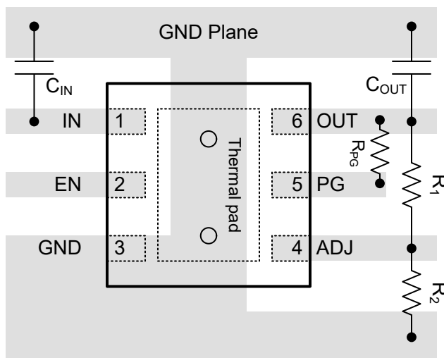
图 7-17. TPS7E67-Q1 DRV 封装的布局示例
