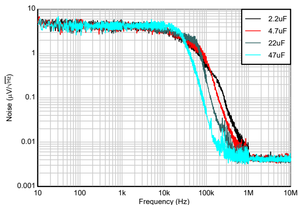
图 5-28. 噪声与 C_{OUT} 间的关系
