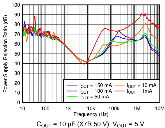
图 5-9. PSRR vs Frequency and I_{OUT}
