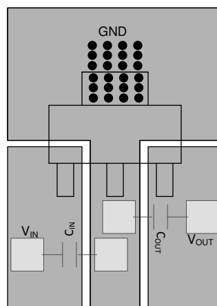
图 10-1. SOT-223 (DCY) Layout
