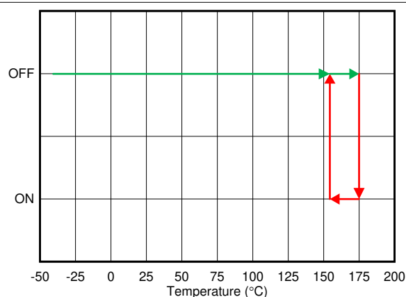
图 6-30. Thermal Shutdown
