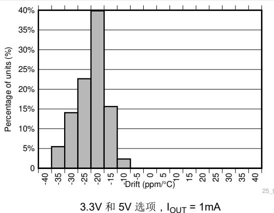
图 5-11. 温漂直方图 ( 25^{\circ}\text{C} 至 150^{\circ}\text{C} )
