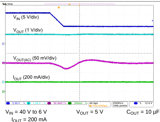
图 18. Line Transient
