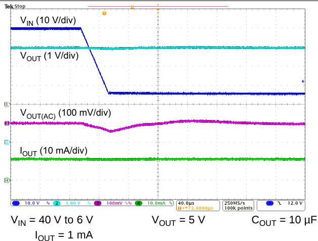
图 16. Line Transient
