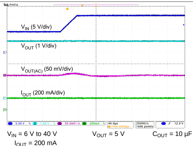
图 17. Line Transient
