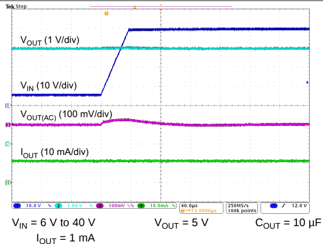
图 15. Line Transient
