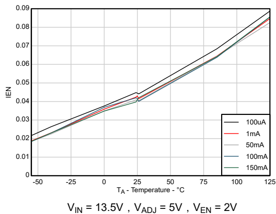
图 5-21. 使能引脚漏电流与环境温度间的关系
