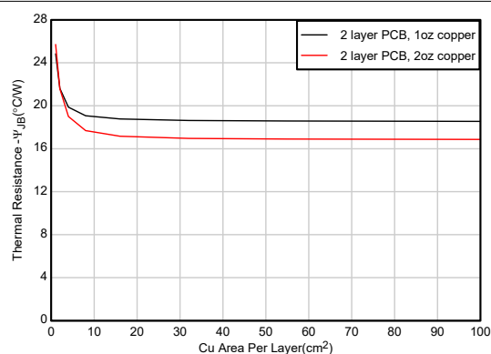
图 7-3. \Psi_{\text{JB}} 与铜面积间的关系 (HSOIC-8 封装, 2 层 PCB)
