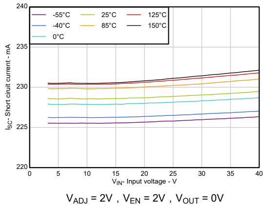
图 5-19. 电流限制与输入电压间的关系
