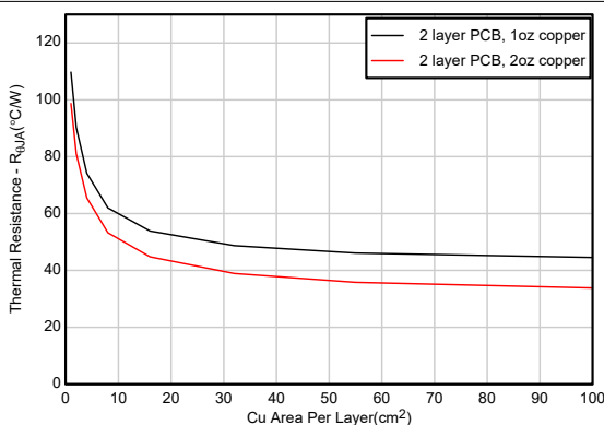
图 7-2. R_{\theta\text{JA}} 与铜面积间的关系 (HSOIC-8 封装, 2 层 PCB)
