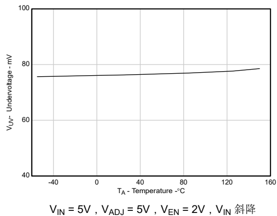
图 5-23. 欠压跳变阈值与环境温度间的关系
