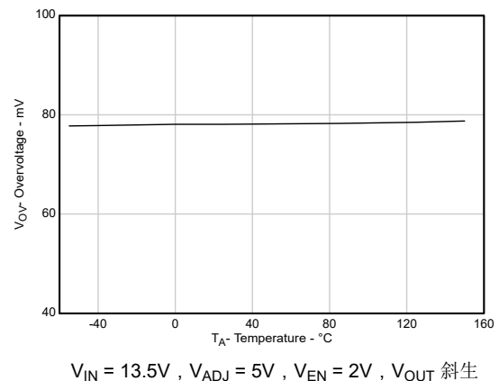
图 5-22. 过压跳变阈值与环境温度间的关系
