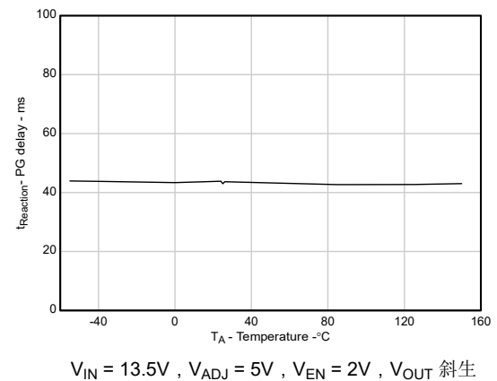
图 5-24. 过压 PG 跳变响应时间与环境温度间的关系
