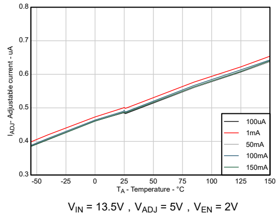
图 5-20. 可调节引脚漏电流与环境温度间的关系
