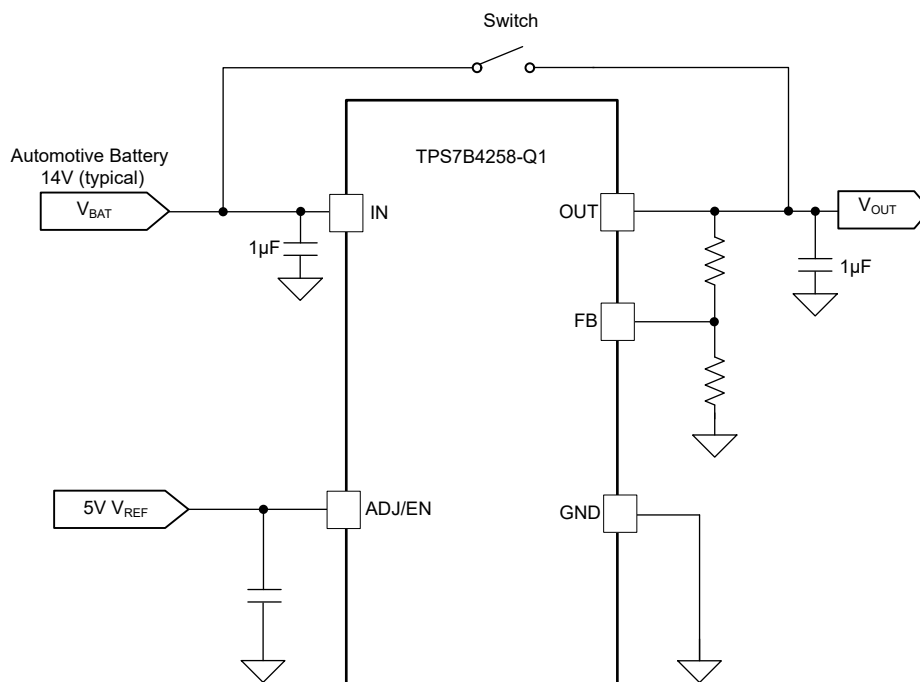
图 6-5. 跟踪器输出对电池短路
