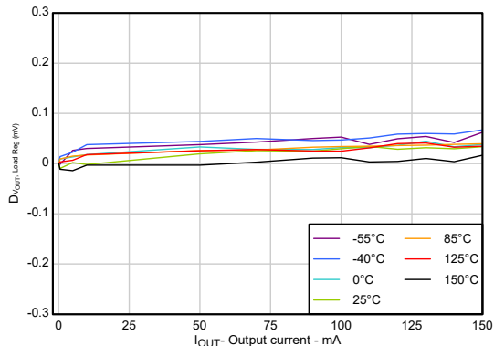
图 5-7. 负载调整率
