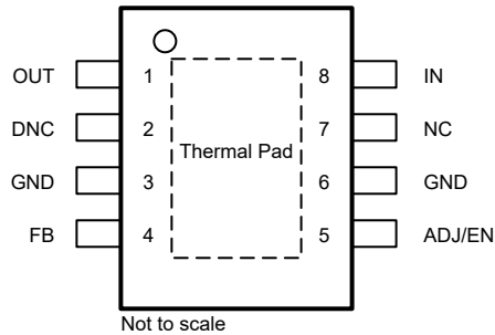
图 4-1. DDA 封装，8 引脚 HSOIC ( 俯视图 )
