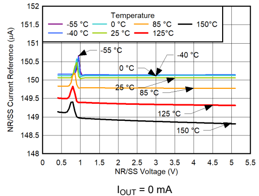
图 6-38. I_{NR/SS} vs V_{NR/SS} and Temperature
