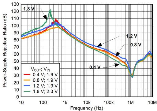
图 6-5. PSRR vs Frequency and Input Pairs
