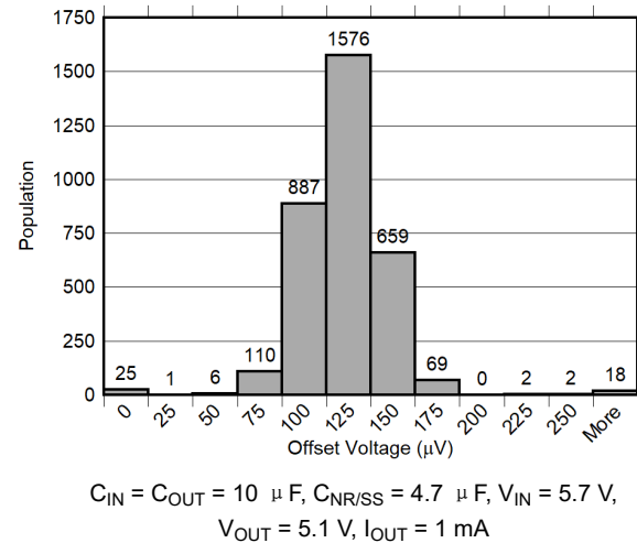
图 6-46. V_{OS} Distribution
