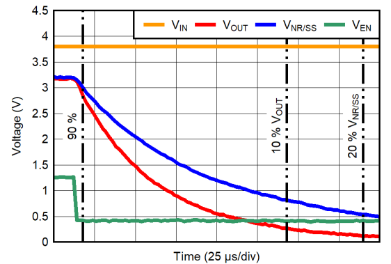
图 6-36. Shutdown Waveform With EN
