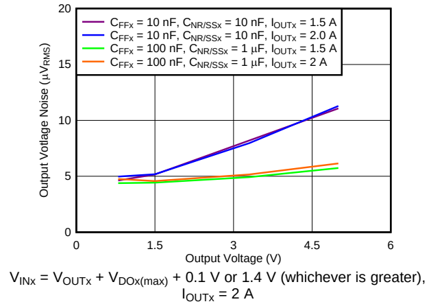
图 8. Output Noise vs Output Voltage
