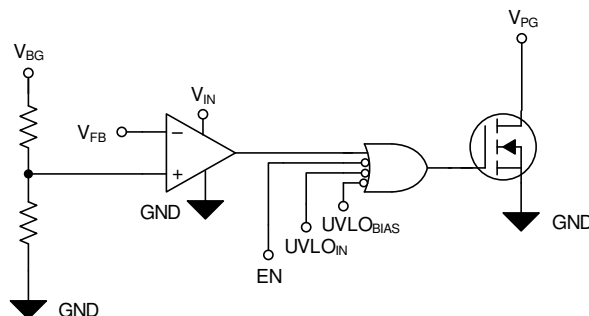
图 7-6. Simplified PG Circuit
