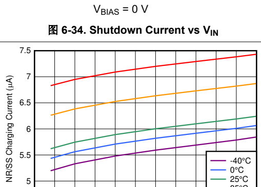
图 6-36. I_{NR/SS} Current vs V_{IN} V_{BIAS} = 0\text{ V}
