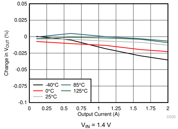
图 7-26. Load Regulation
