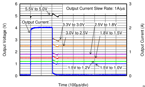
具有七种不同输出的负载瞬态响应
