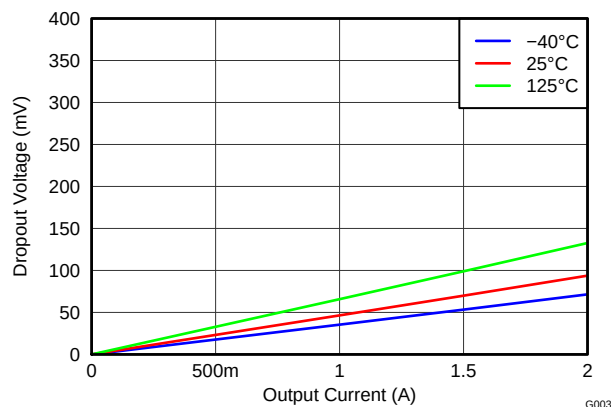
压降与输出电流间的关系 ( V_{OUT} = 3.3V )
